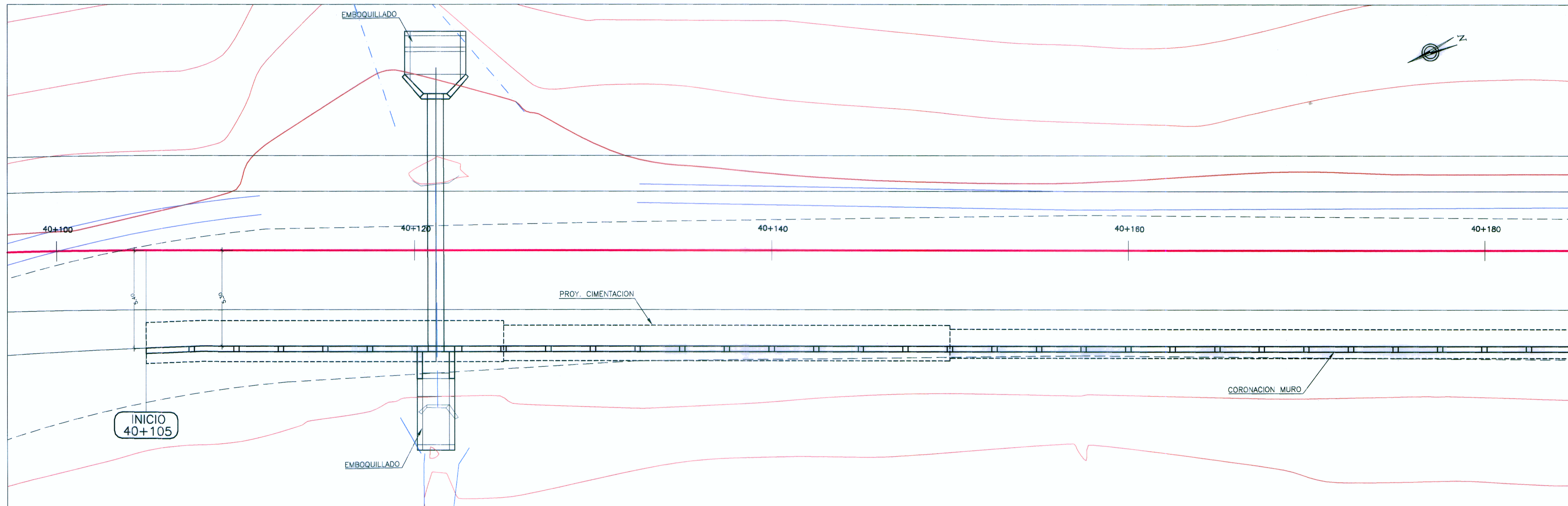
PLANTA ESC.: 1/125
