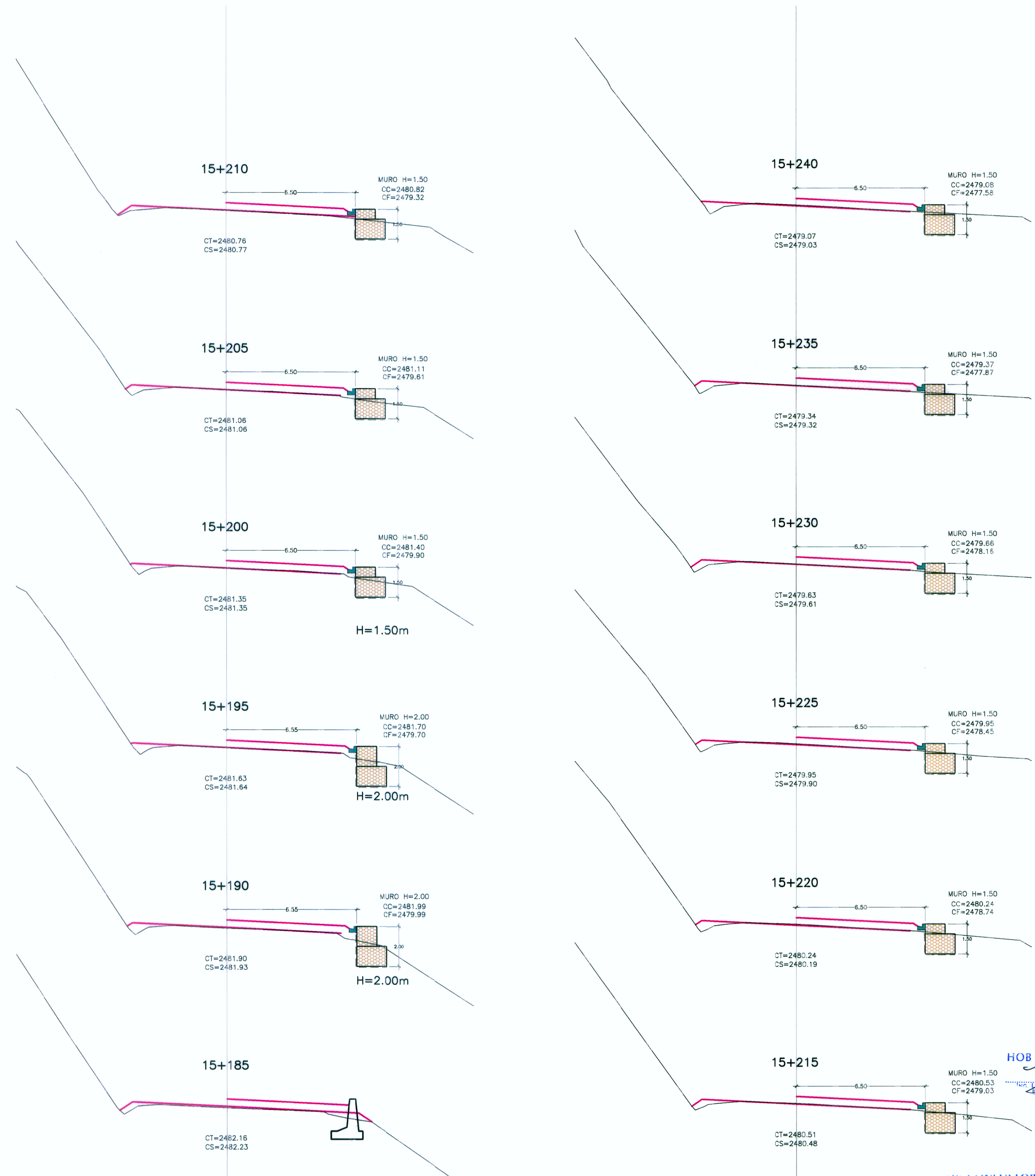
SECCIONES TRANSVERSALES ESC.: 1/125
