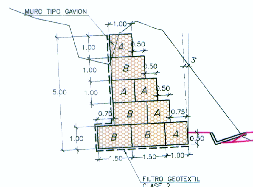
DETALLE MURO GAVION ESC. 1/100
