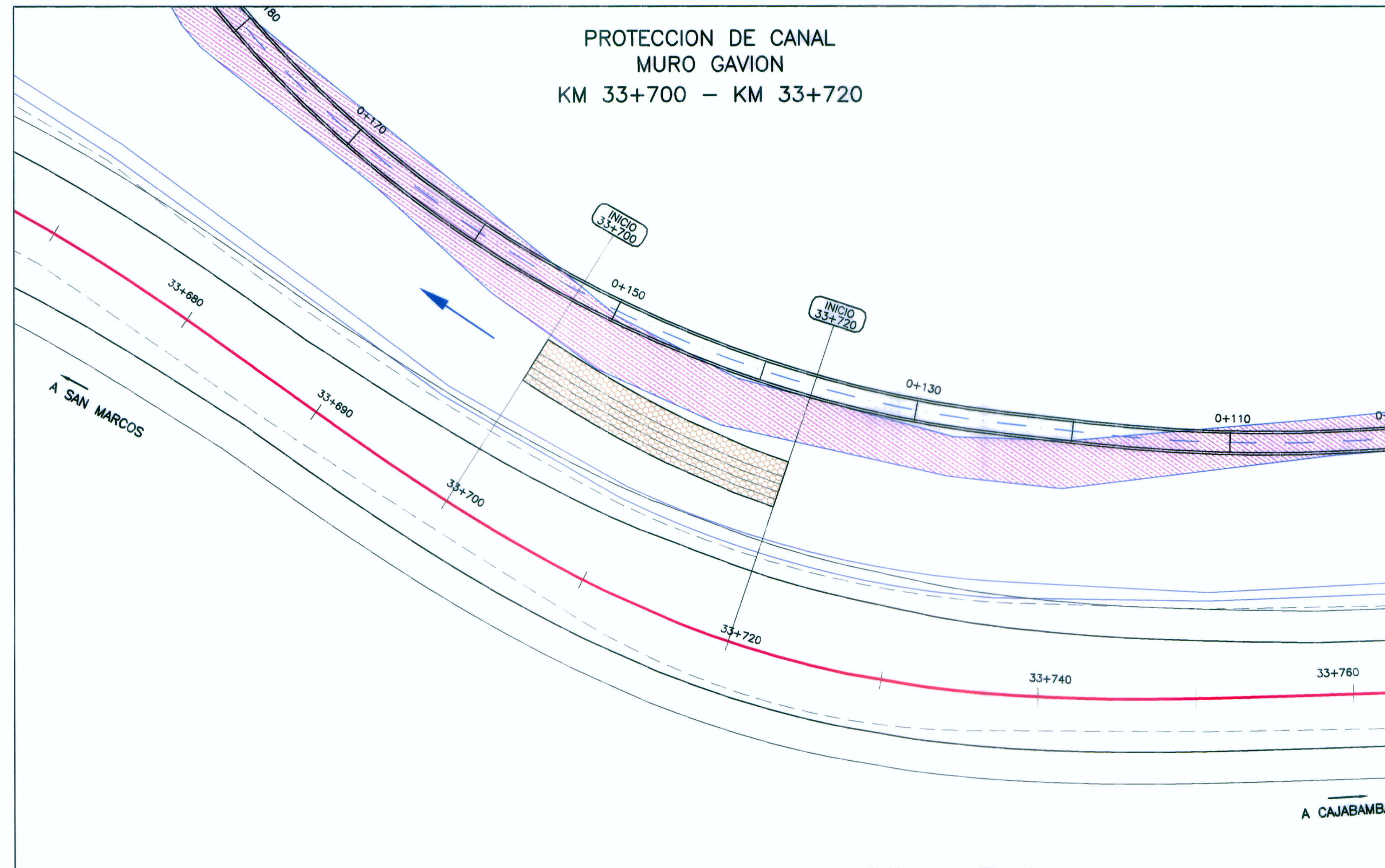
PLANTA ESC. 1/200
