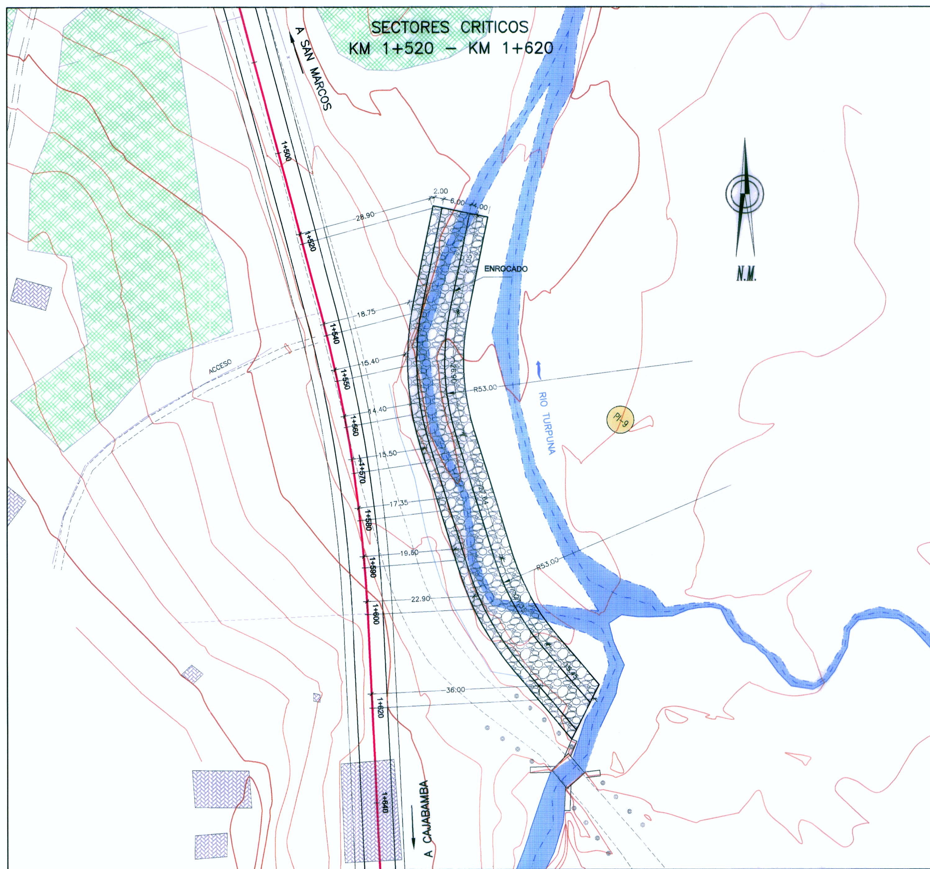
PLANTA ESC. 1:500
