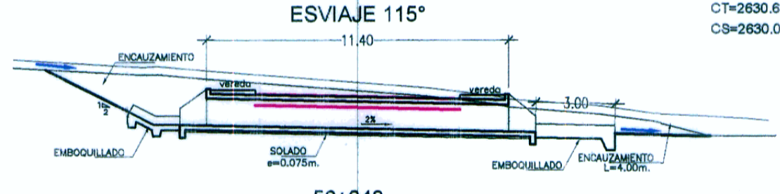
ALCANTARILLA TIPO MC 1.00x1.00m PROYECTAR 56+643.40 ESVIAJE 115°
