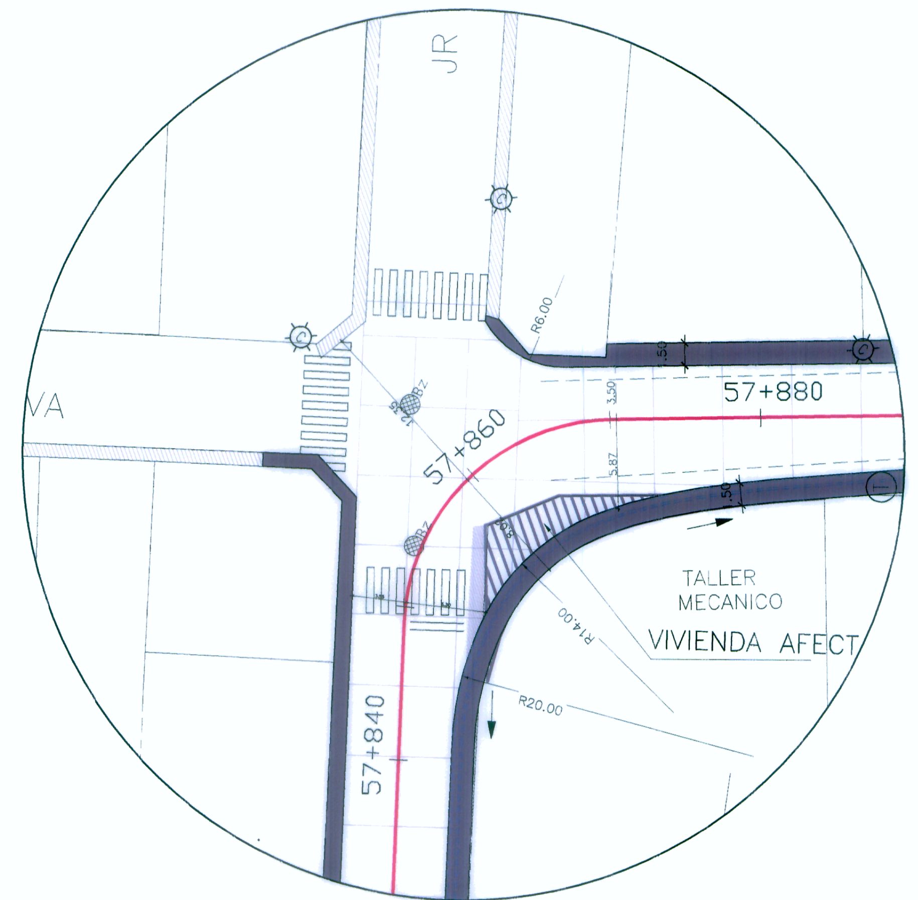
DETALLE 1 ESC. 1/250
