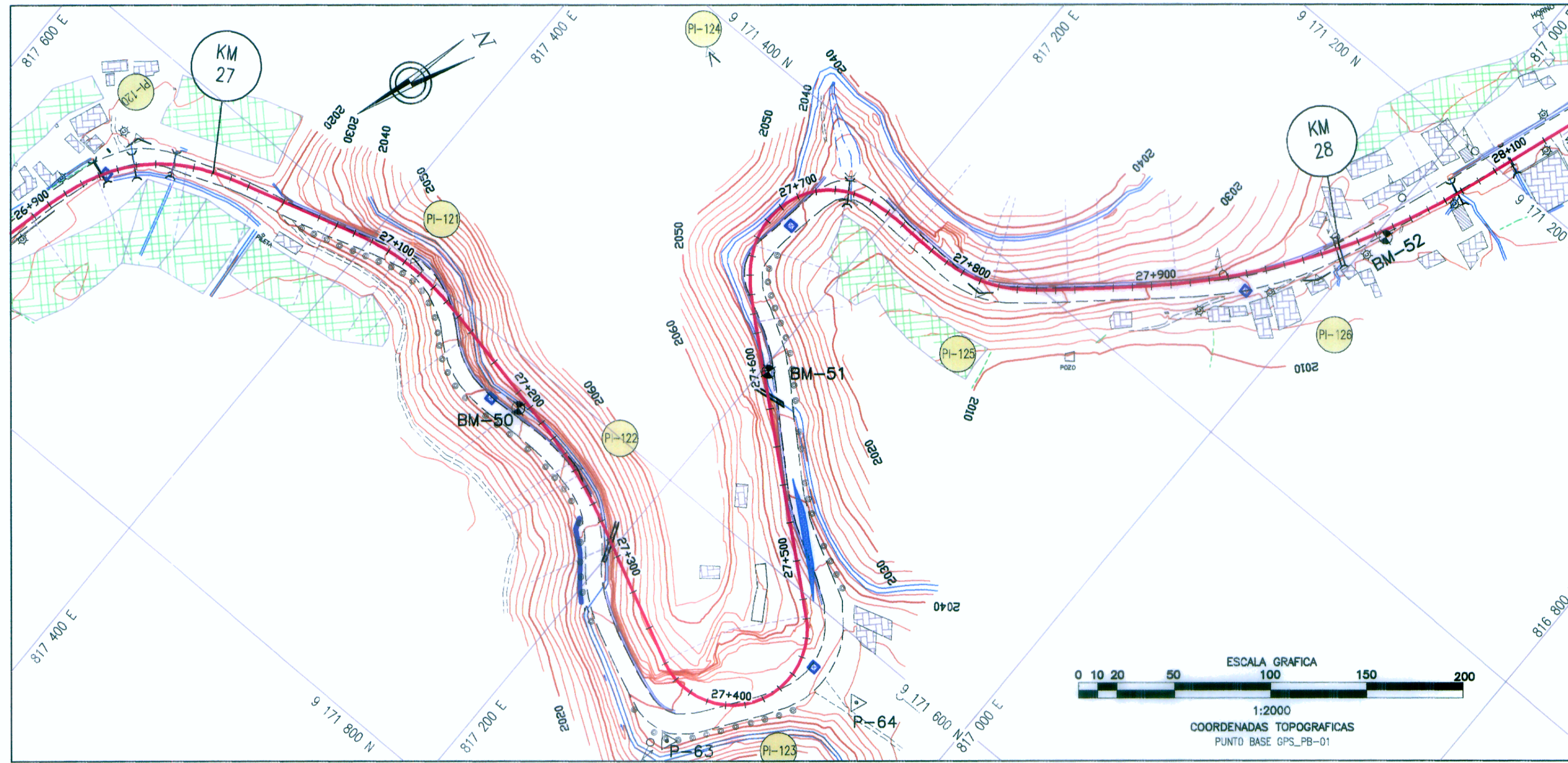
PLANTA 1:2000
