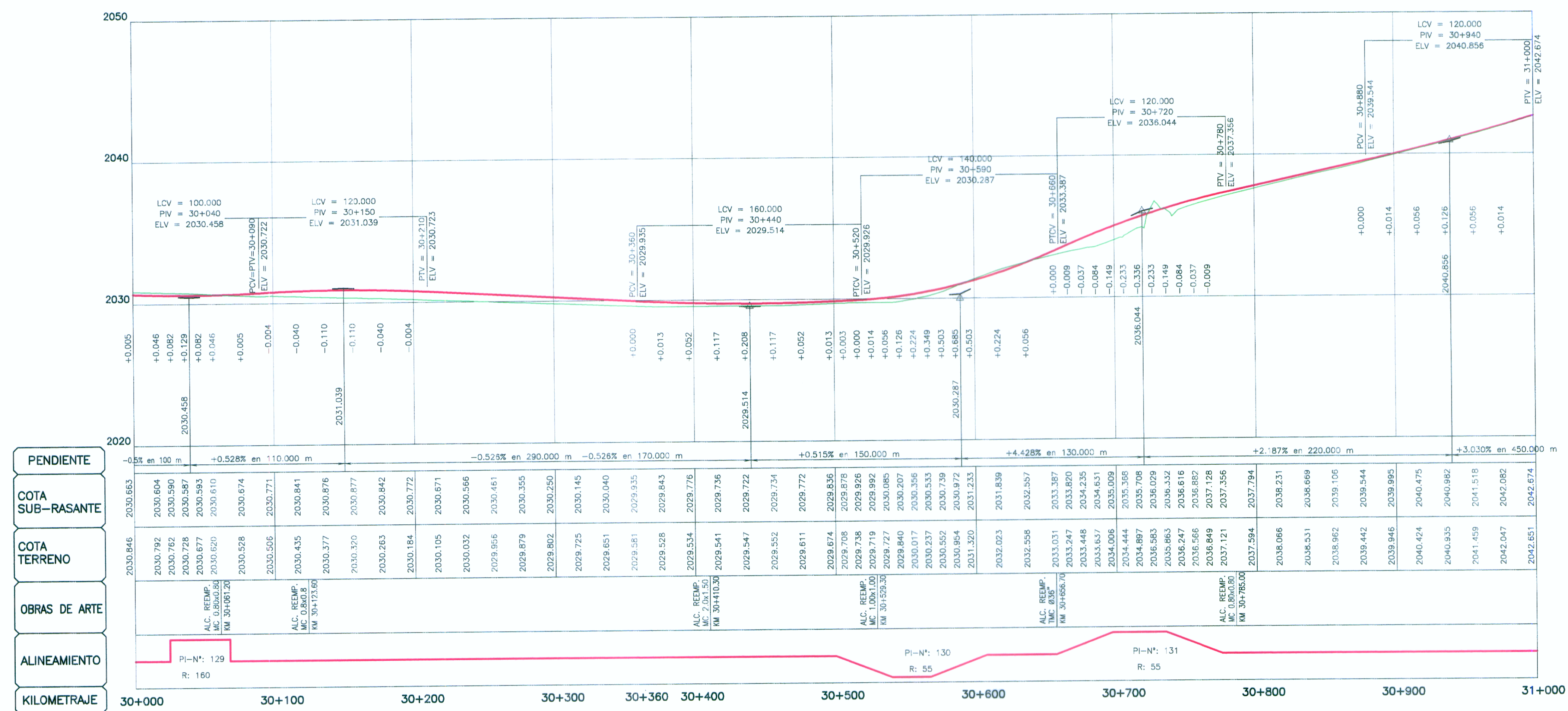
PERFIL LONGITUDINAL H=1:2000 V=1:200
