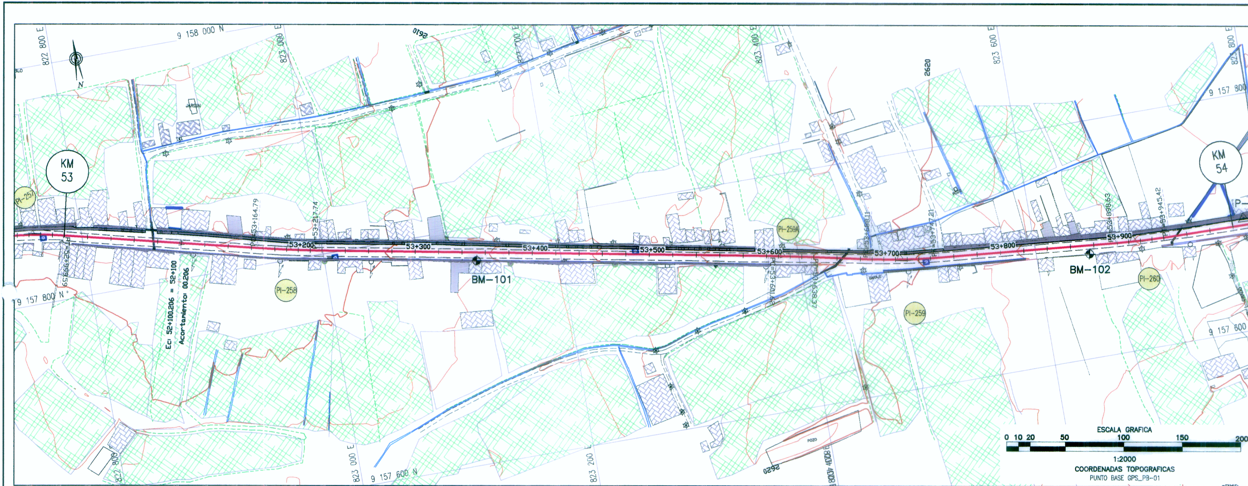
PLANTA 1:2000
