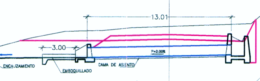
ALCANTARILLA TIPO TMC ø36" PROYECTAR 1+650
