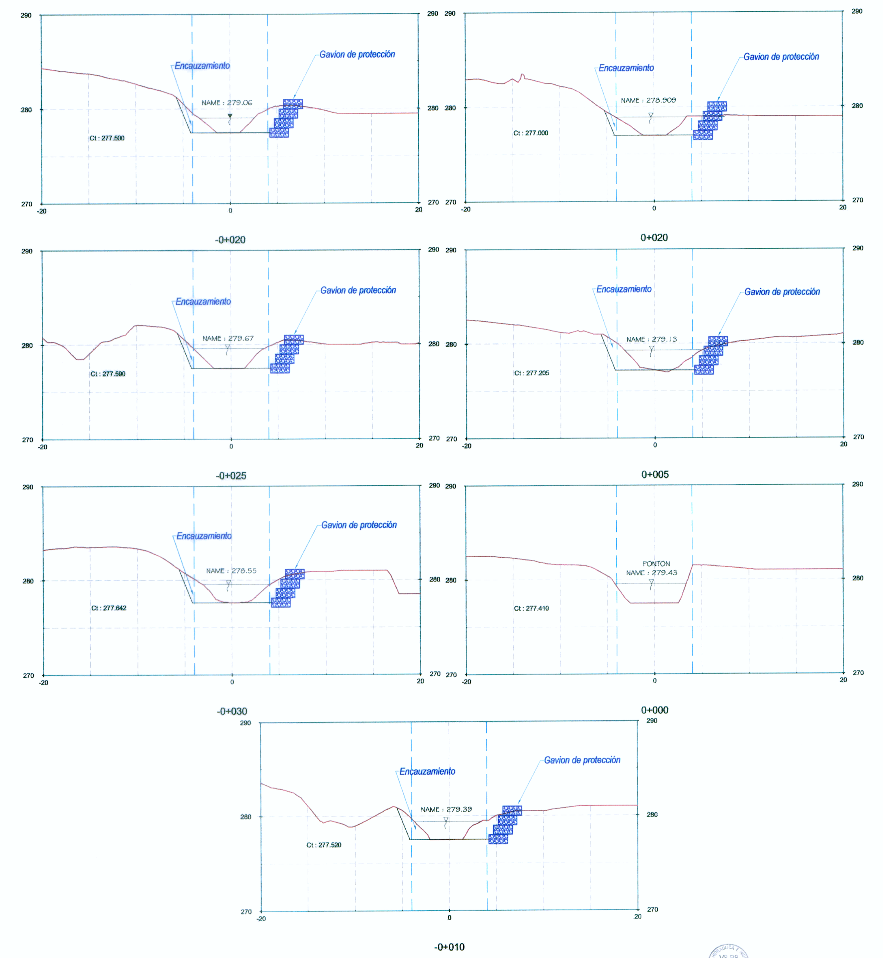
SECCIONES Esc. 1/250
