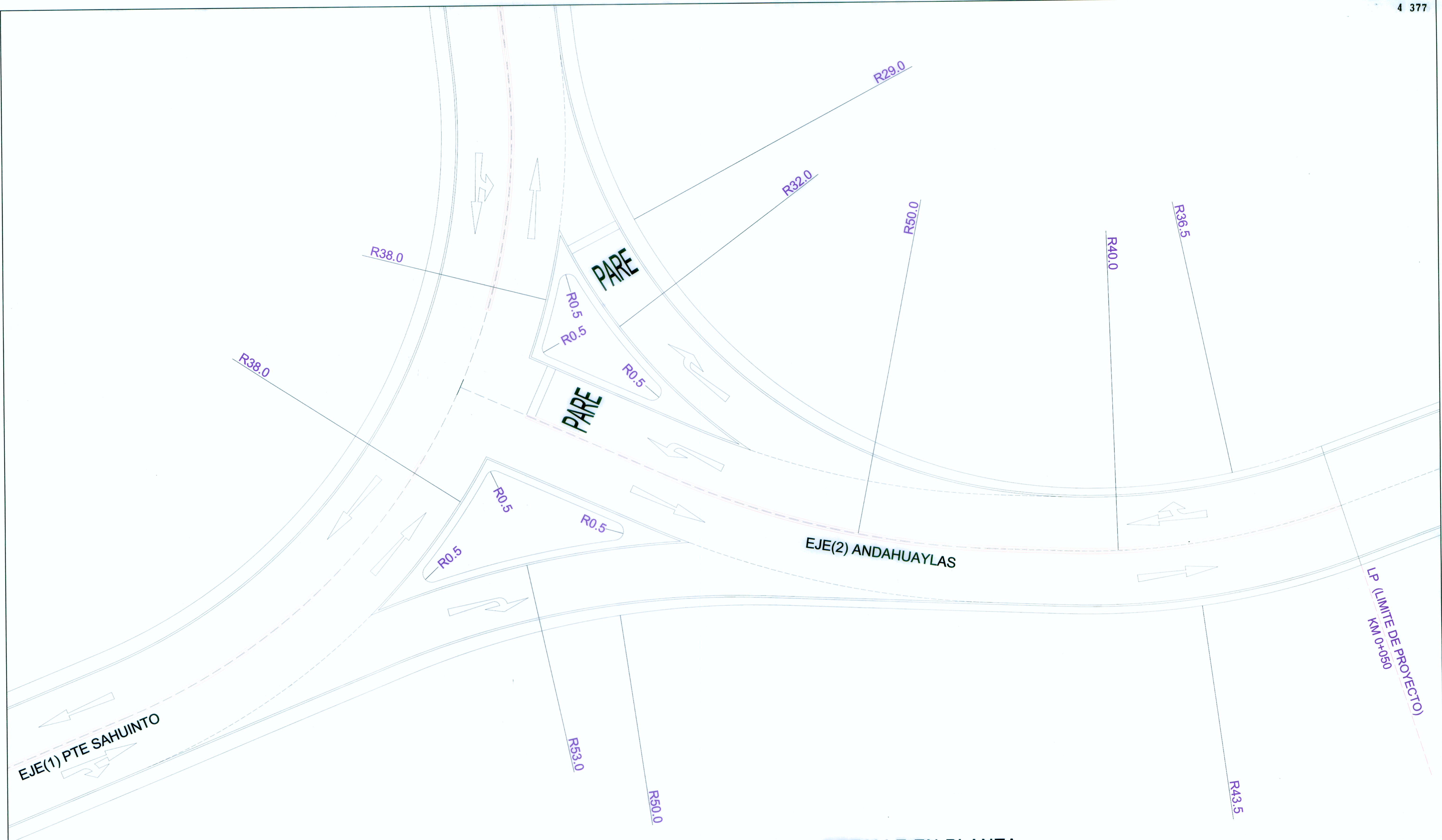
DETALLE EN PLANTA ESC. 1/200
