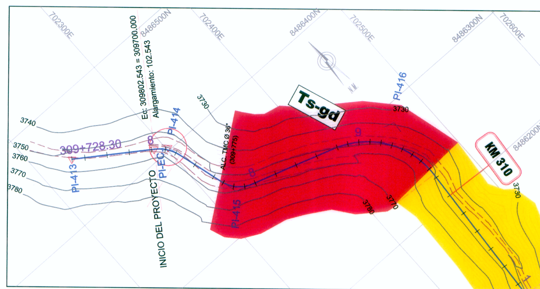
PLANTA Esc. 1/4000
