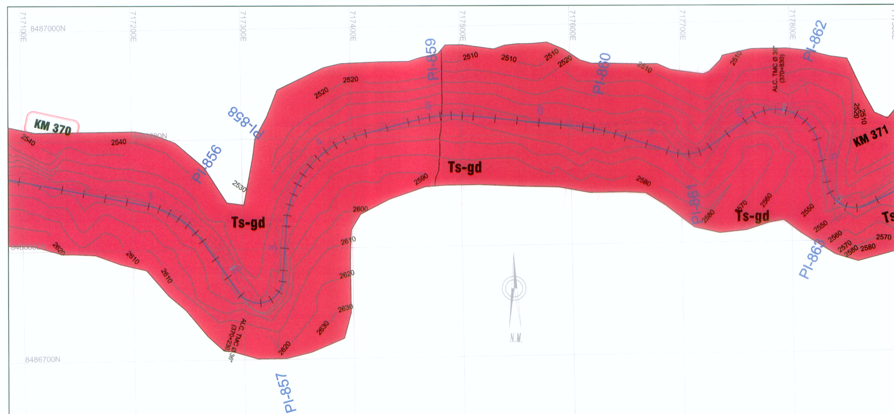
PLANTA Esc. 1/4000
