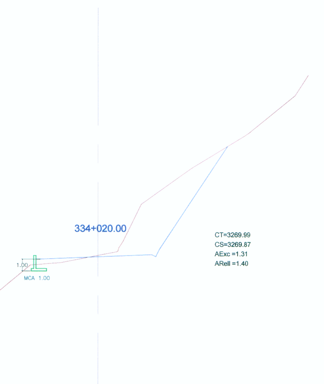
18 MURO DE CONTENCION KM. 334+015 - KM. 334+025
