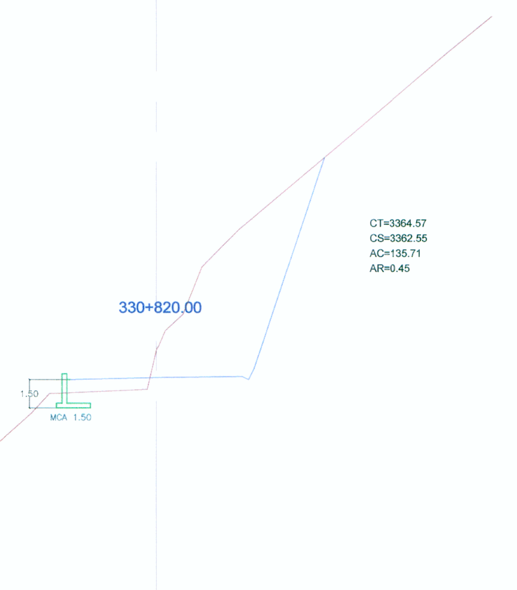
17 MURO DE CONTENCION KM. 330+815 - KM. 330+825
