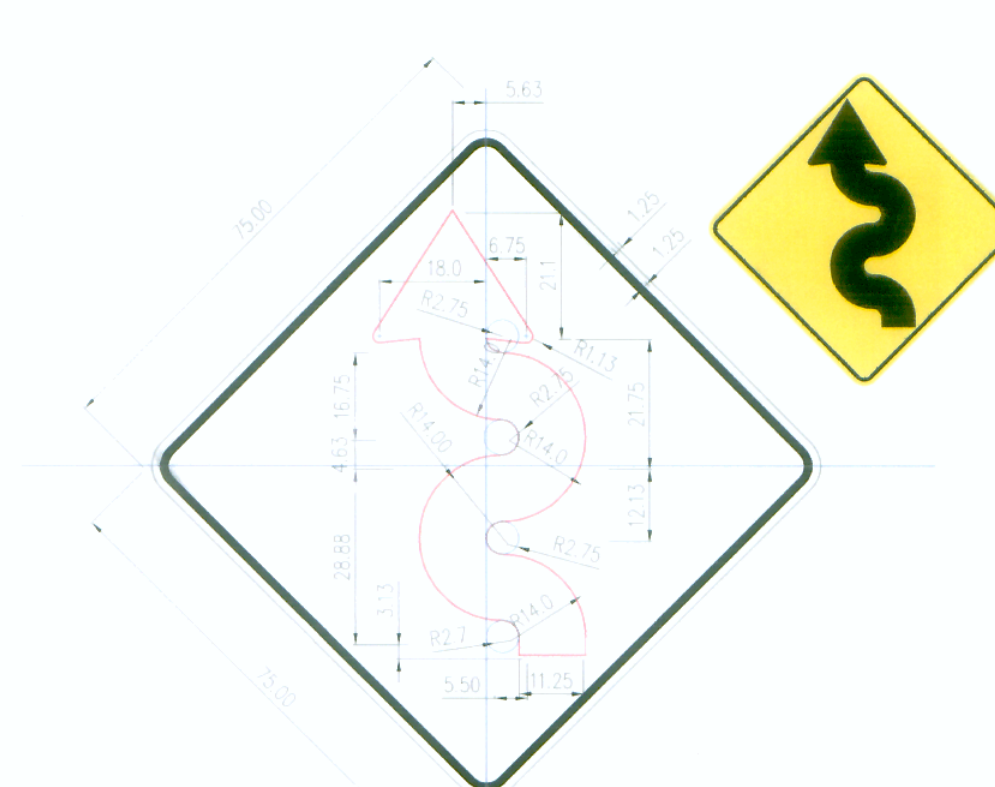
P-5-1B CAMINO SINUOSO (IZQUIERDA)
