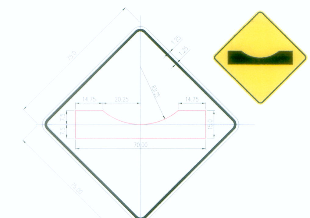
P-34 BADEN O DEPRESION
