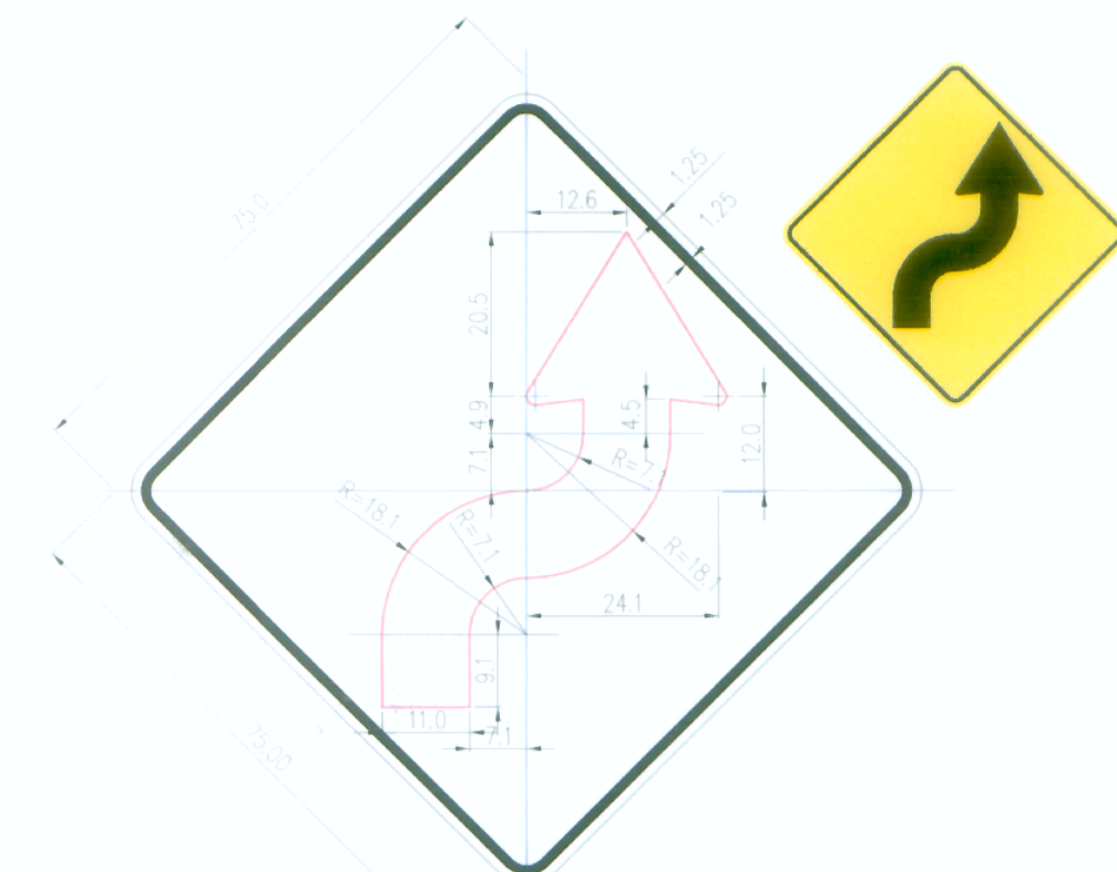
P-4A CURVA Y CONTRA CURVA (D-I)
