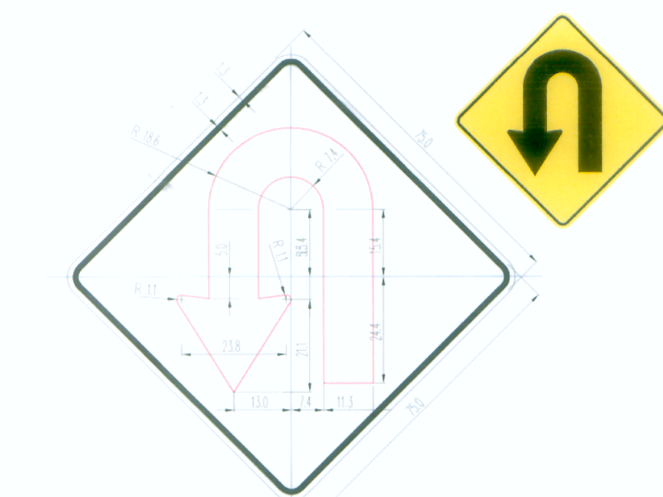
P-5-2 B CURVA EN U - IZQUIERDA
