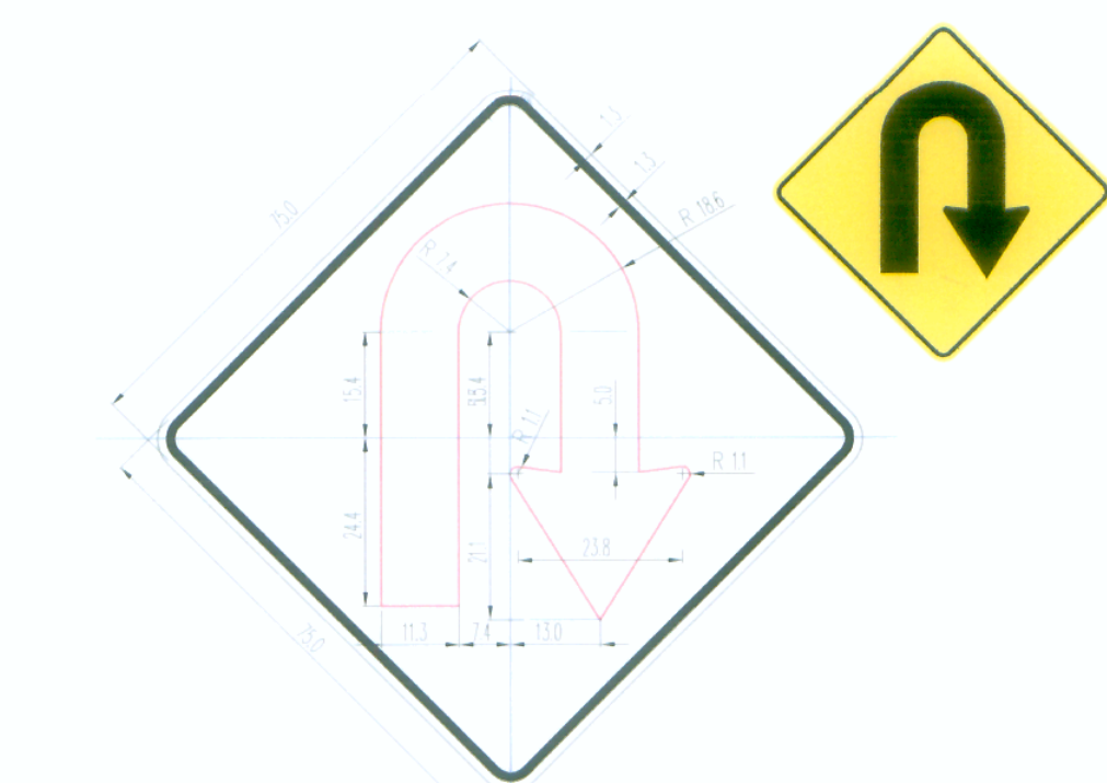
P-5-2 A CURVA EN U - DERECHA
