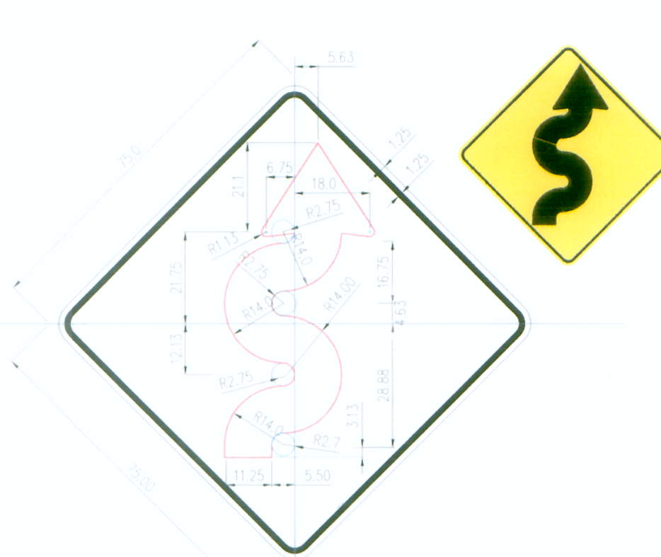
P-5-1A CAMINO SINUOSO (DERECHA)
