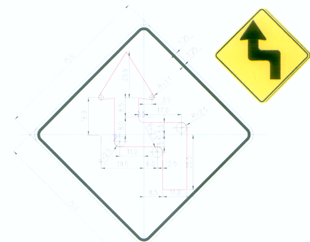
P-3B CURVA Y CONTRA CURVA PRONUNCIADA (I-D)
