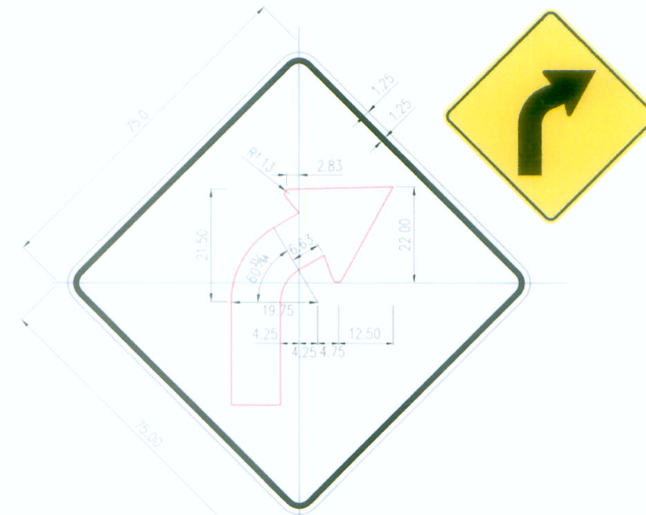
P-2A CURVA A LA DERECHA
