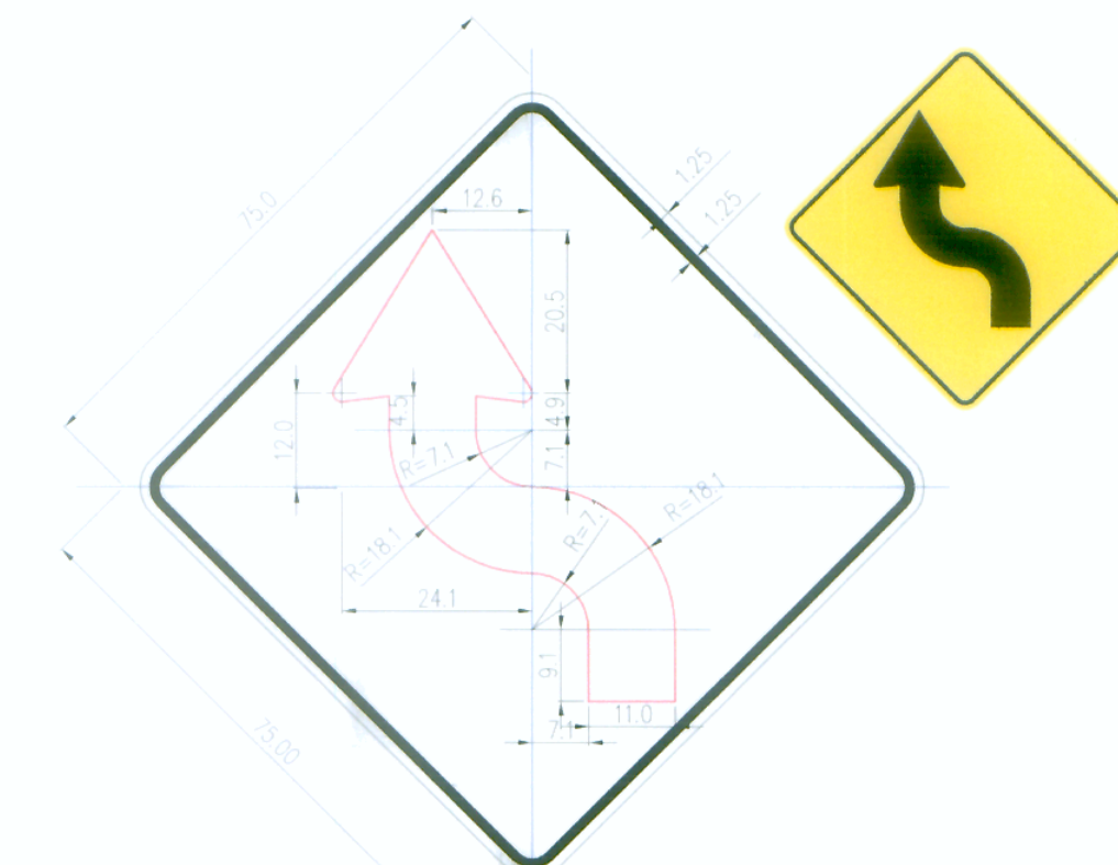
P-4B CURVA Y CONTRA CURVA (I-D)
