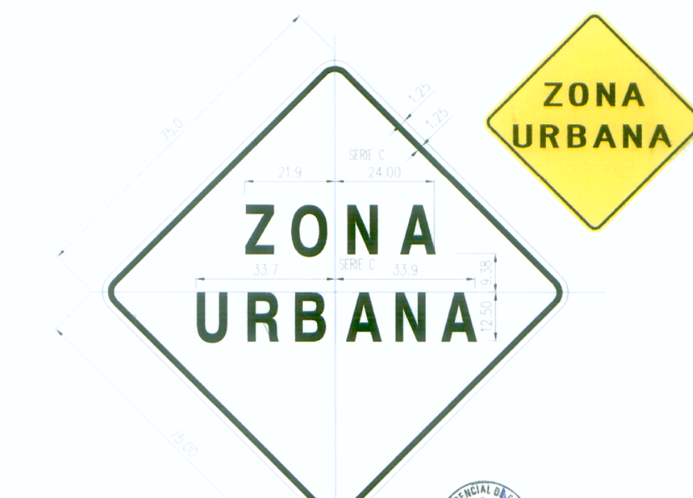
P-56 ZONA URBANA
