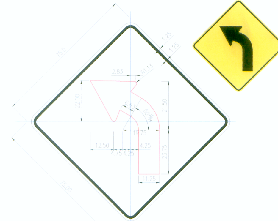
P-2B CURVA A LA IZQUIERDA
