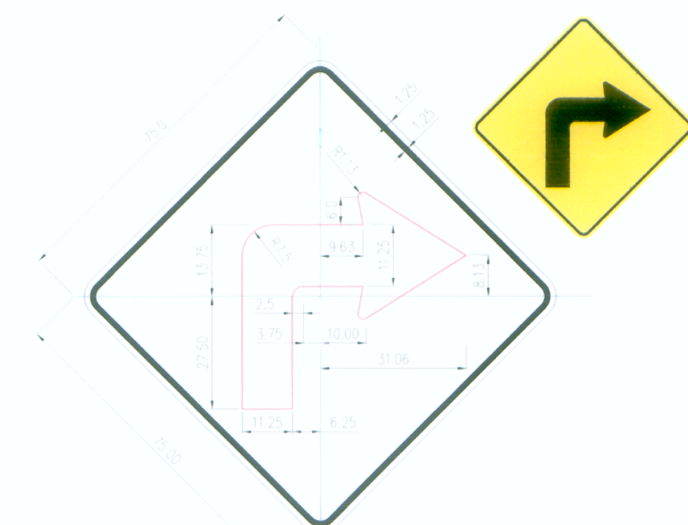
P-1A CURVA PRONUNCIADA A LA DERECHA
