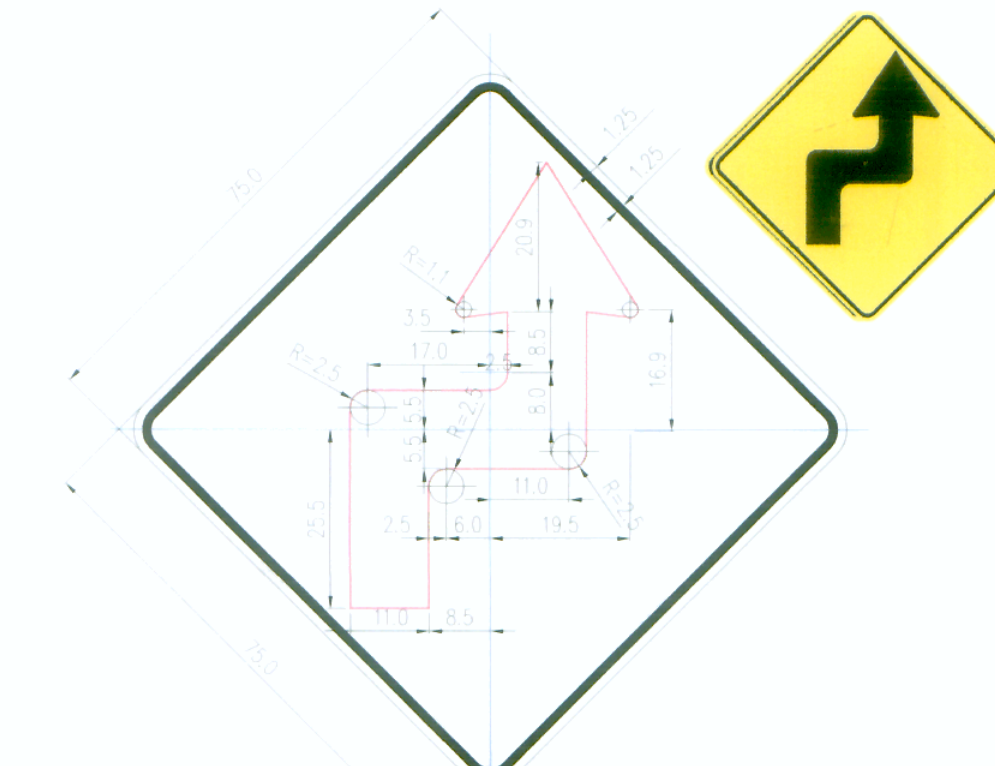
P-3A CURVA Y CONTRA CURVA PRONUNCIADA (D-I)
