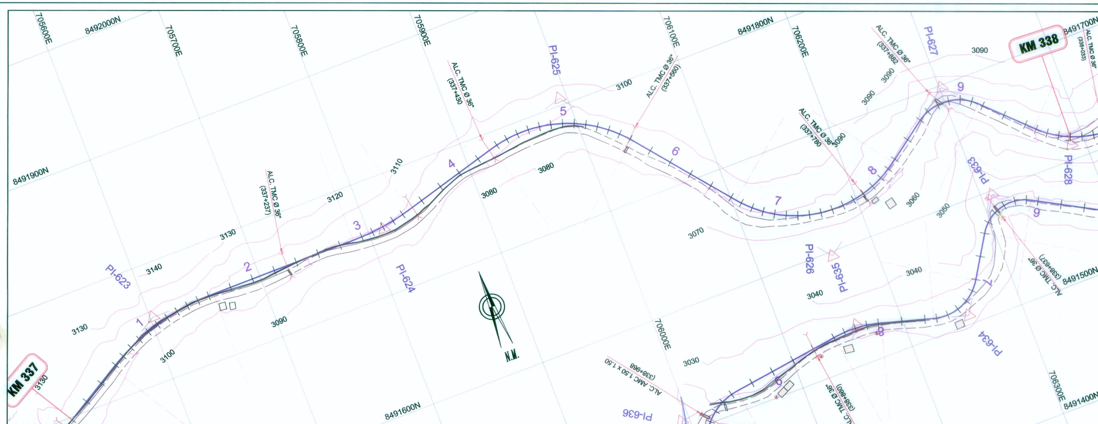
PLANTA Esc. 1/4000
