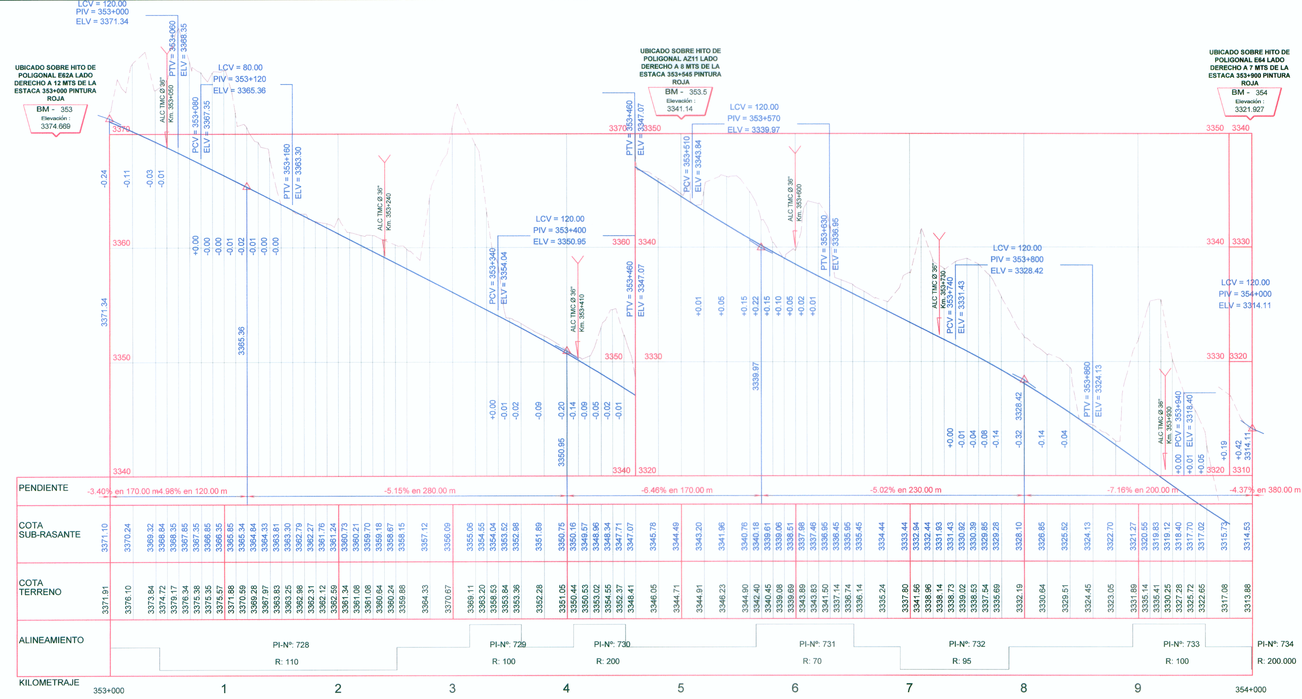
PERFIL LONGITUDINAL Esc. Hor.: 1/4000 Esc. Ver.: 1/400
