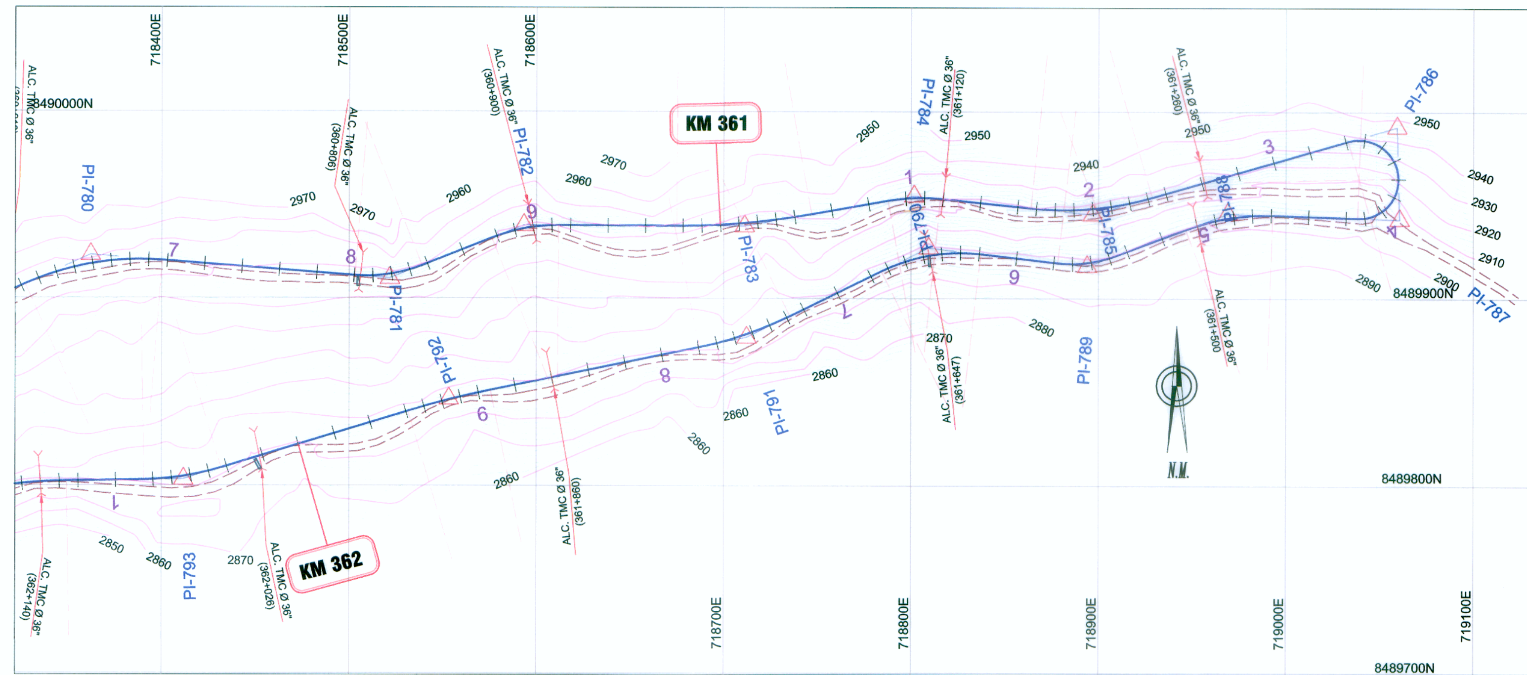
PLANTA Esc. 1/4000
