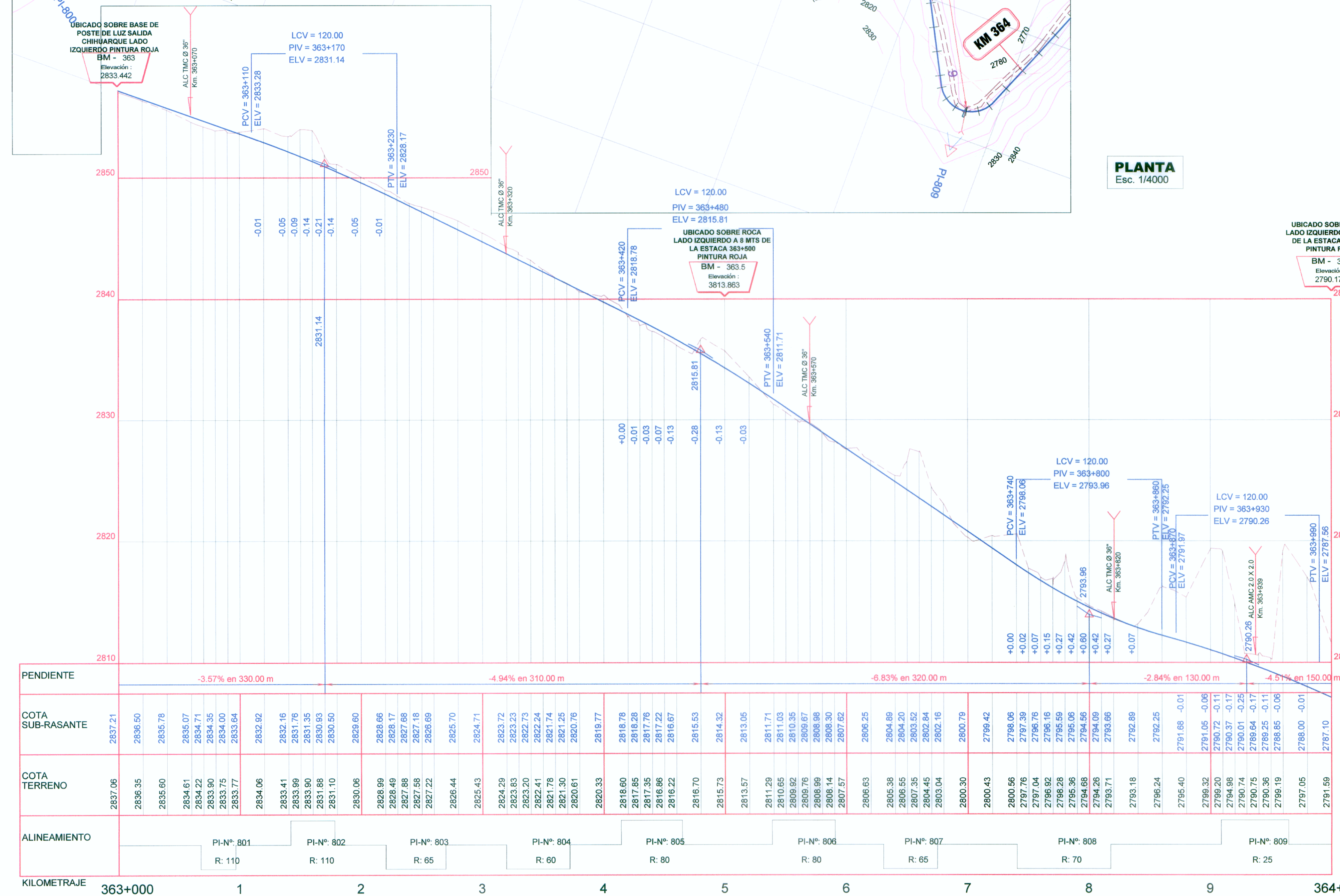
PERFIL LONGITUDINAL Esc. Hor. : 1/4000 Esc. Ver. : 1/400
