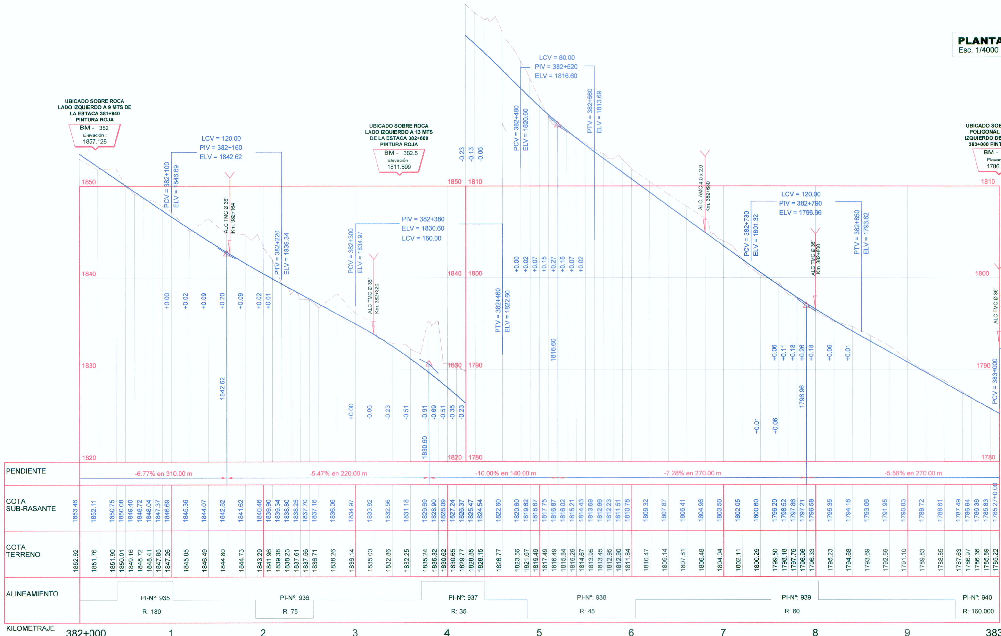
PERFIL LONGITUDINAL Esc. Hor.: 1/4000 Esc. Ver.: 1/400
