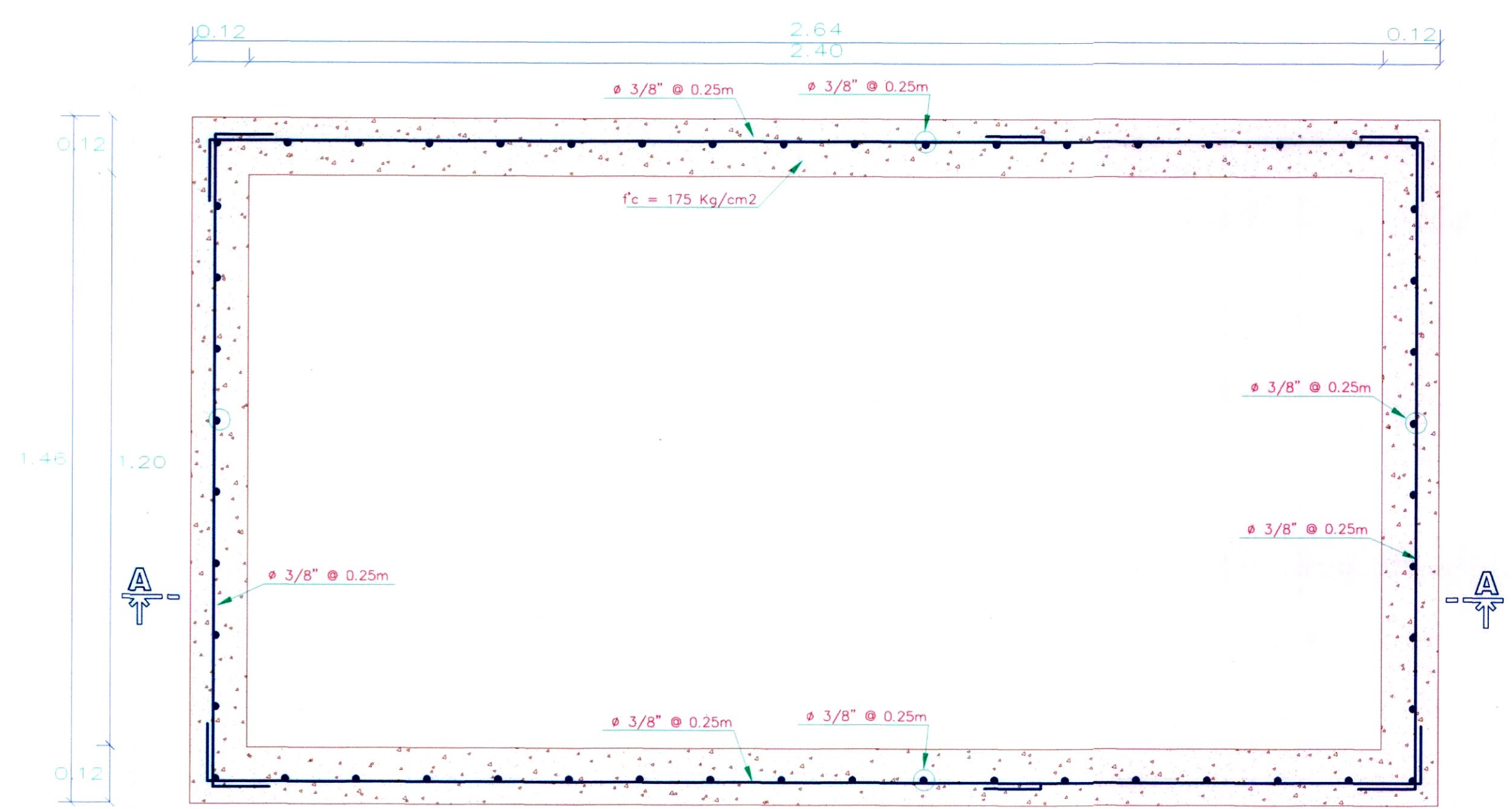
PLANTA ESTRUCTURAL CISTERNA ESC. ---1/10
