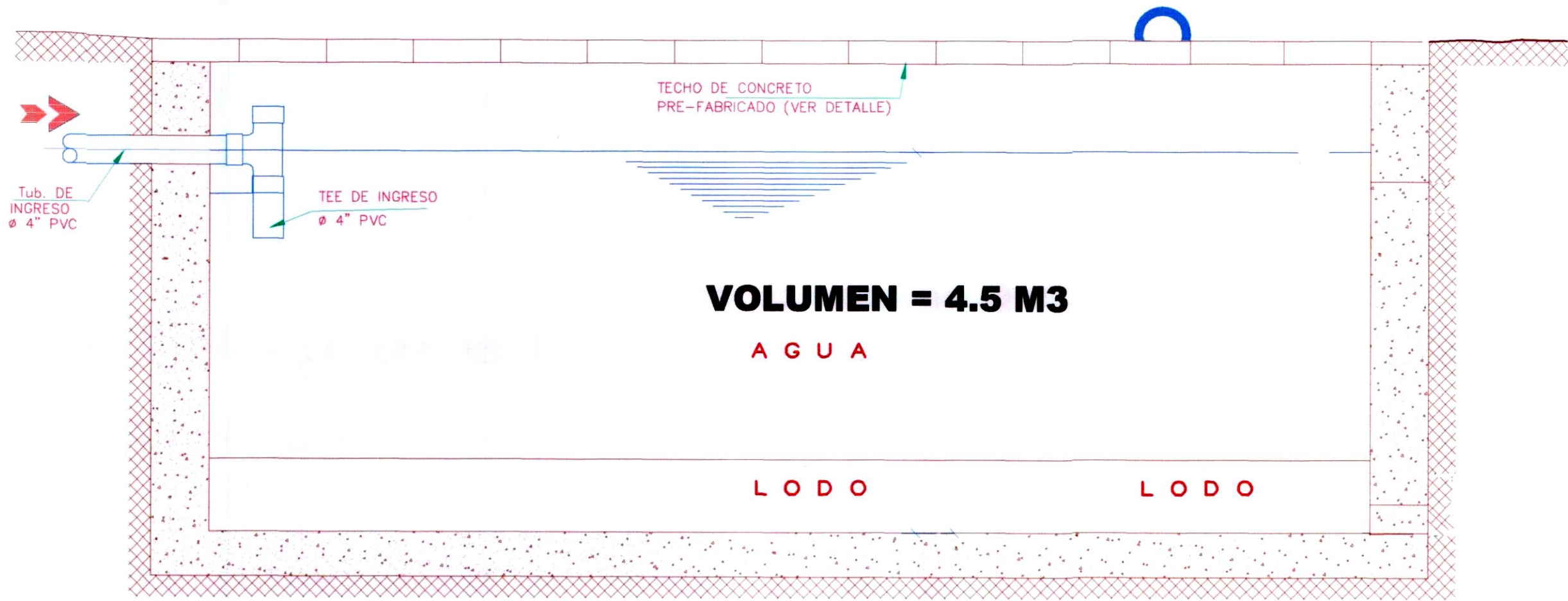
CORTE A - A ESC. ---1/10
