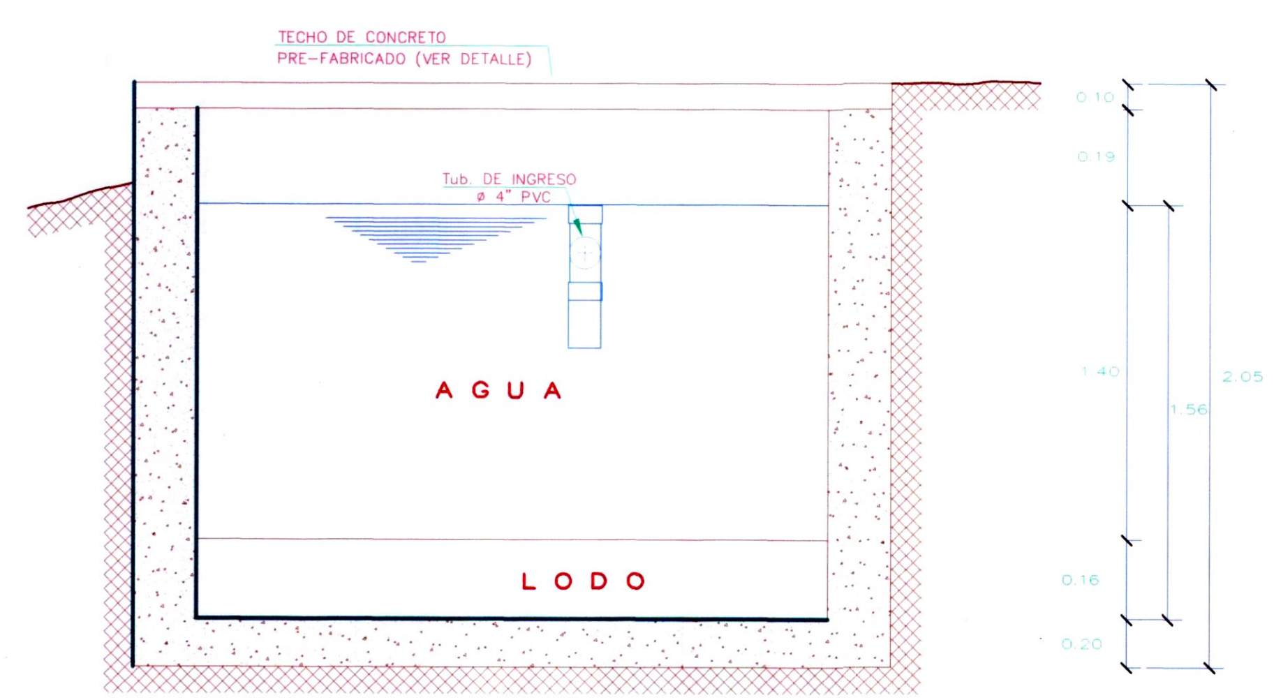
CORTE B - B ESC. ---1/10
