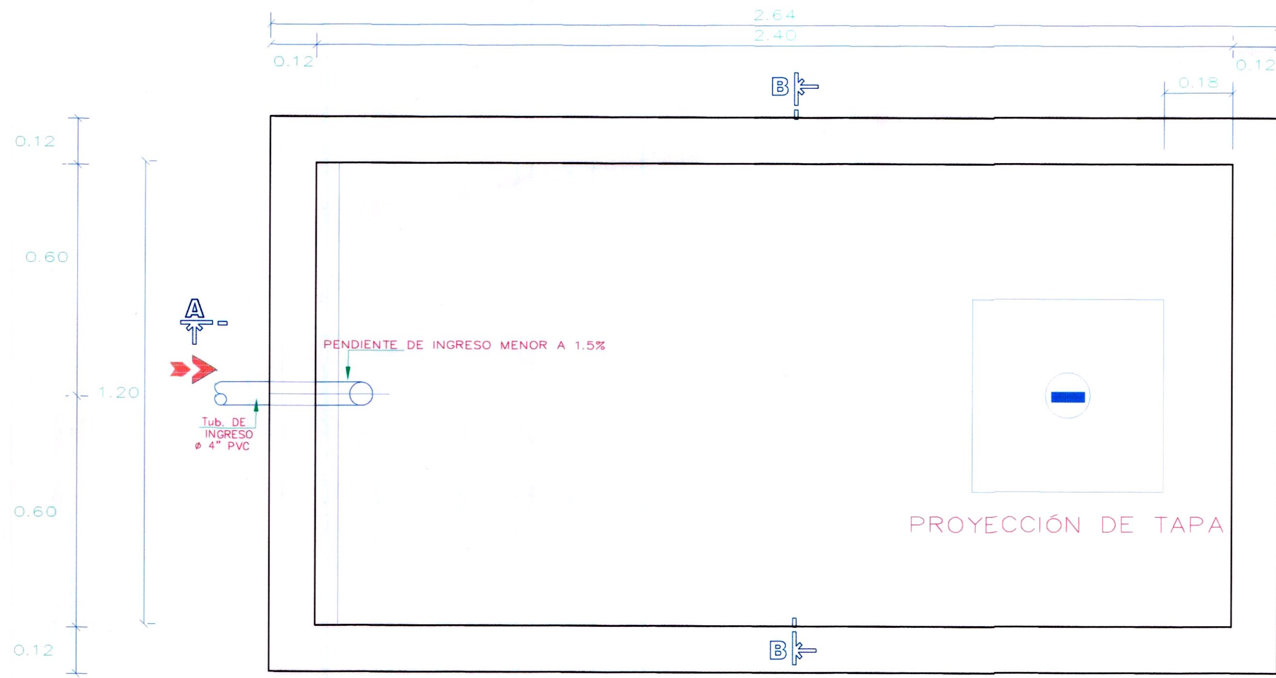
PLANTA CISTERNA ESC. ---1/10
