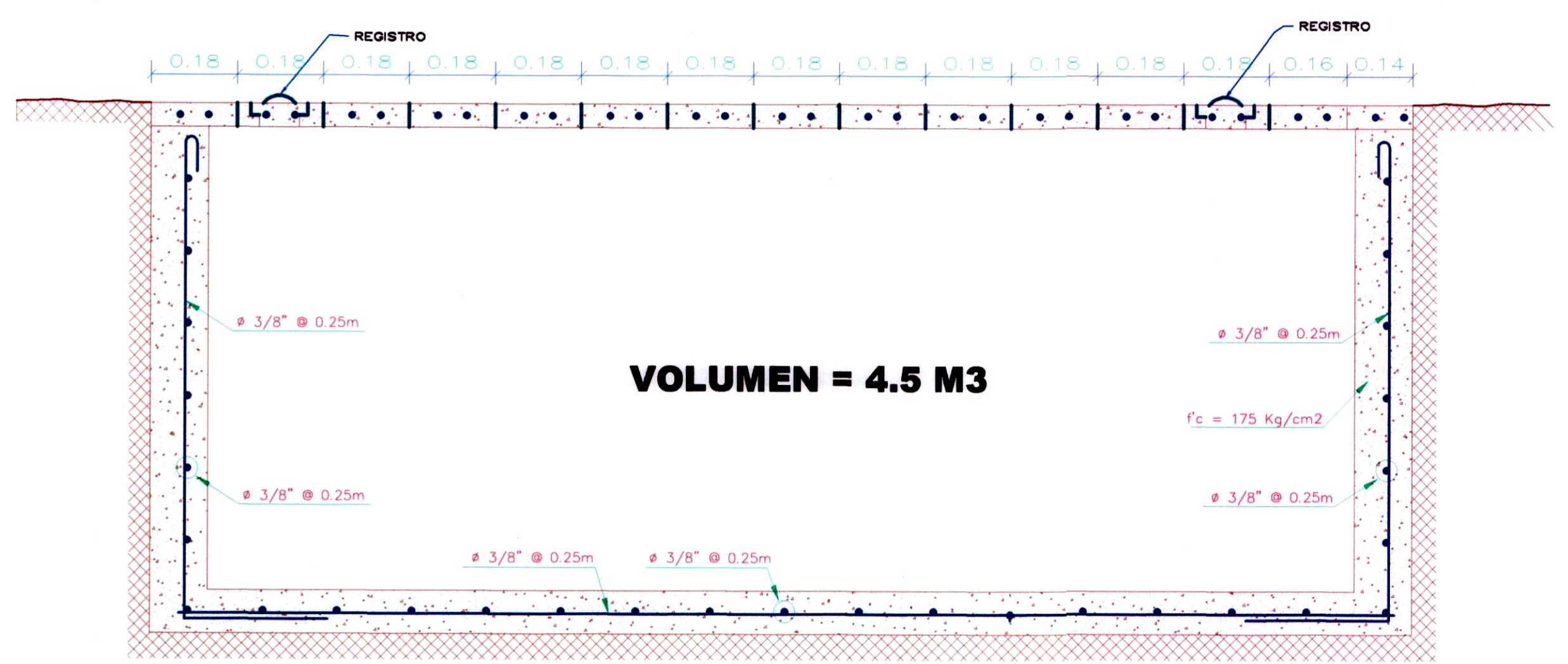
CORTE ESTRUCTURAL A-A ESC. ---1/10
