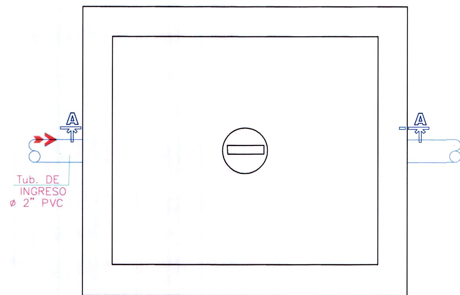
PLANTA TRAMPA DE GRASA ESC. -----1/5
