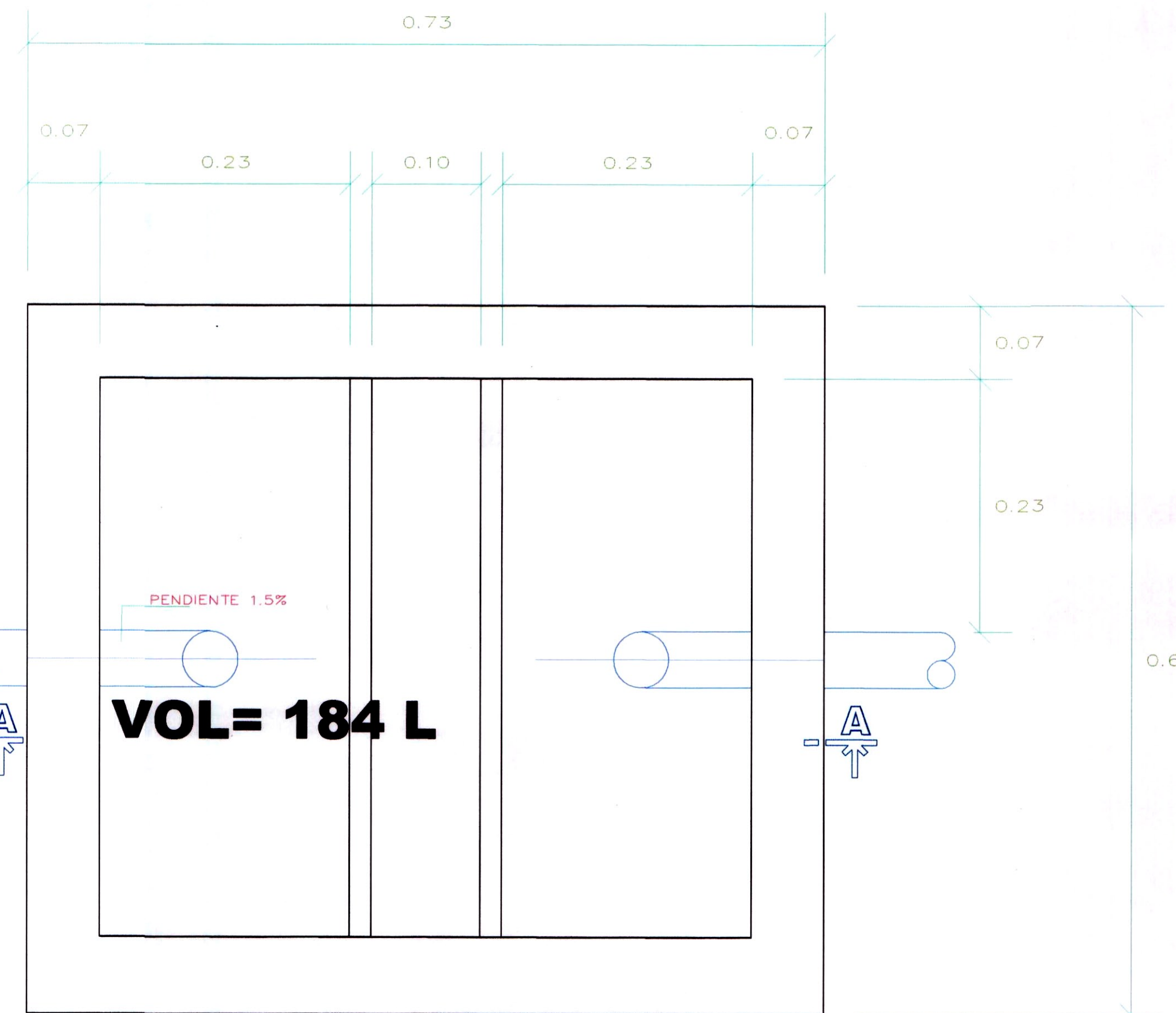
PLANTA TRAMPA DE GRASA ESC. -----1/10
