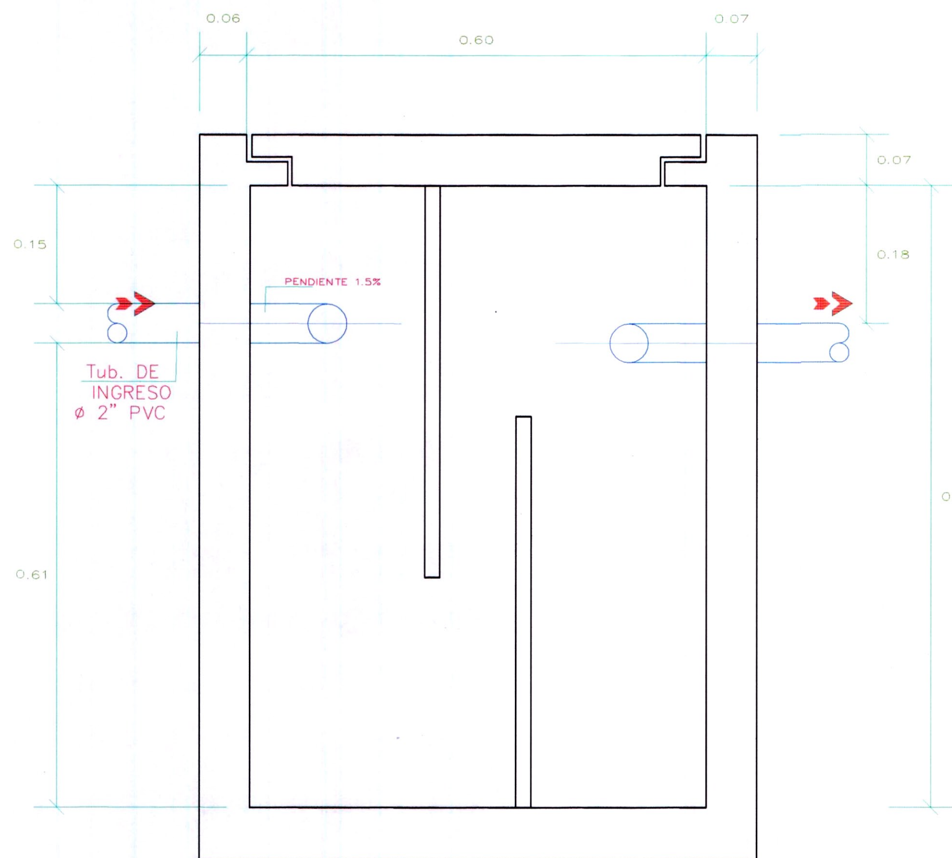
CORTE A - A ESC. -----1/5
