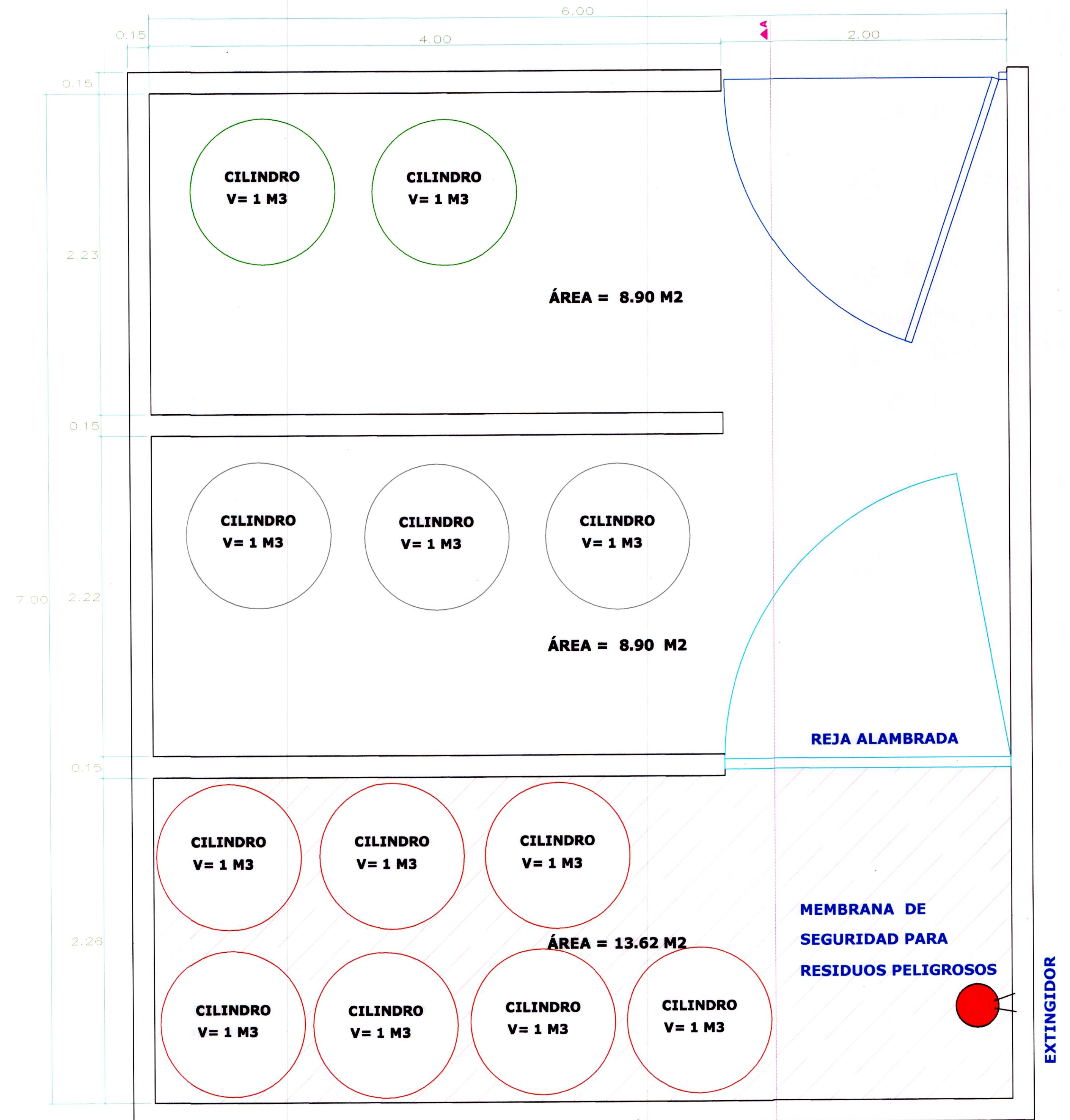
PLANTA BLOQUE SANITARIO ESC. ----1/20
