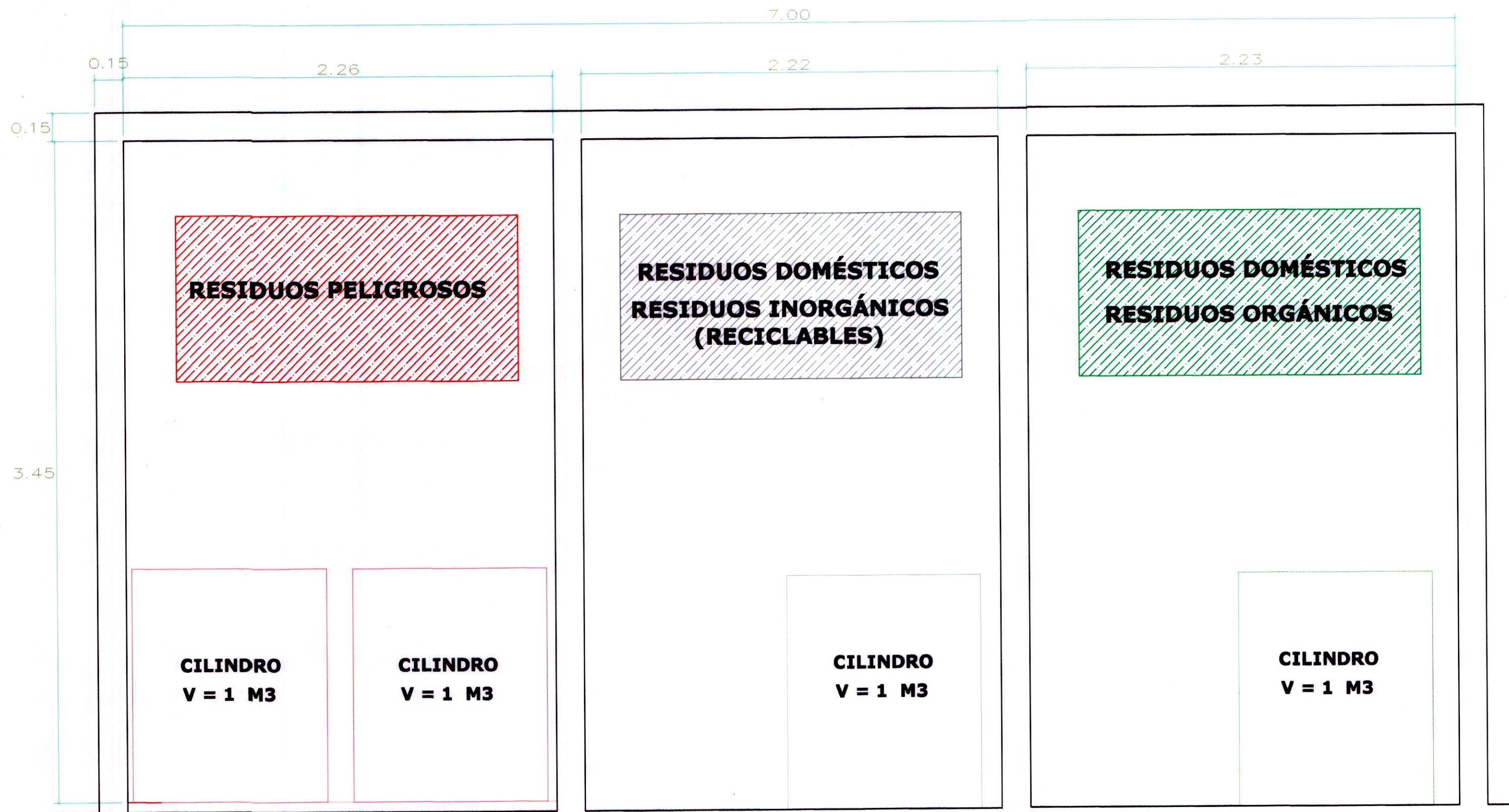
CORTE A-A BLOQUE SANITARIO ESC. ----1/20
