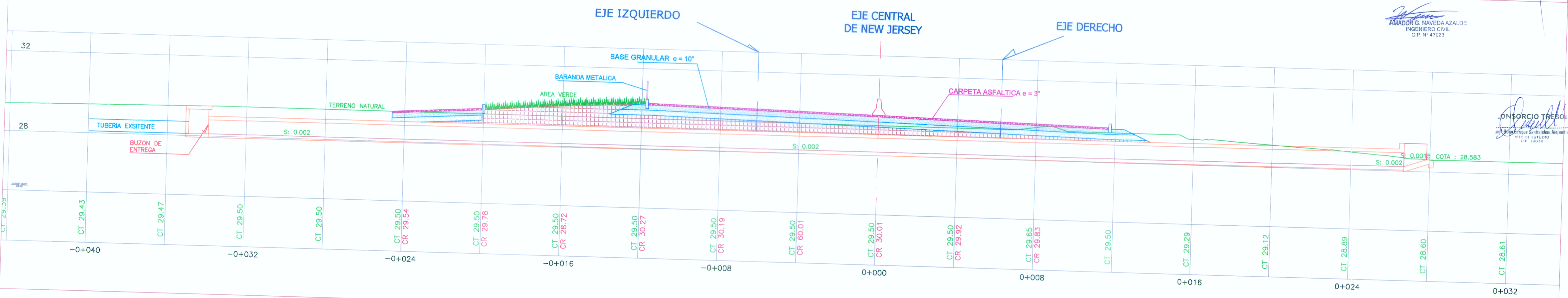
PERFIL LONGITUDINAL
