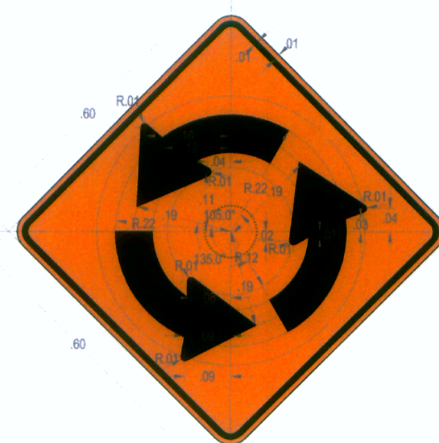
P-15 ROTONDA ESC: 1/10
