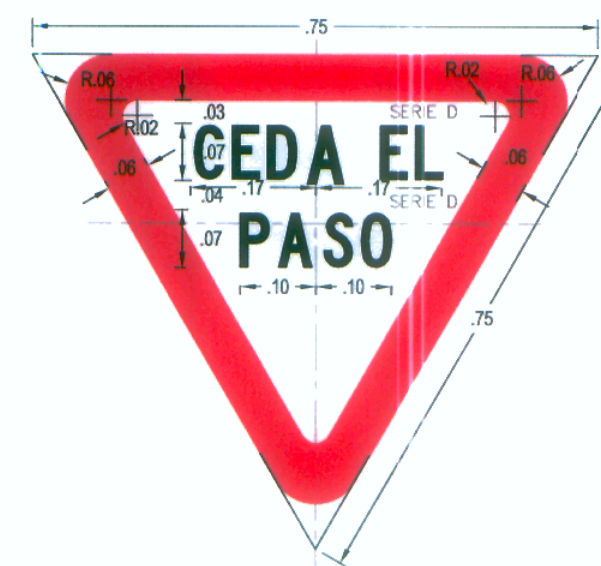
R-2 CEDA EL PASO ESC: 1/10
