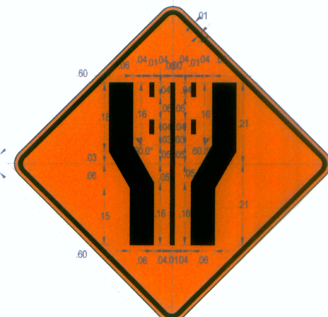
P-22 ENSANCHE DE LA CALZADA ESC: 1/10
