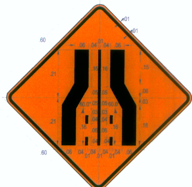
P-18 REDUCCION DE LA CALZADA ESC: 1/10
