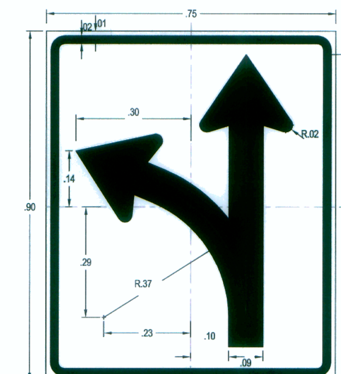
R-5-2 CARRIL PERMITIDO PARA VOLTEO Y PARA SEGUIR DE FRENTE ESC: 1/10
