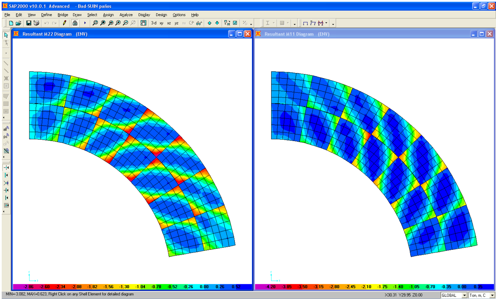
MOMENTOS MIN. DIRECCIONES 1 Y 2
