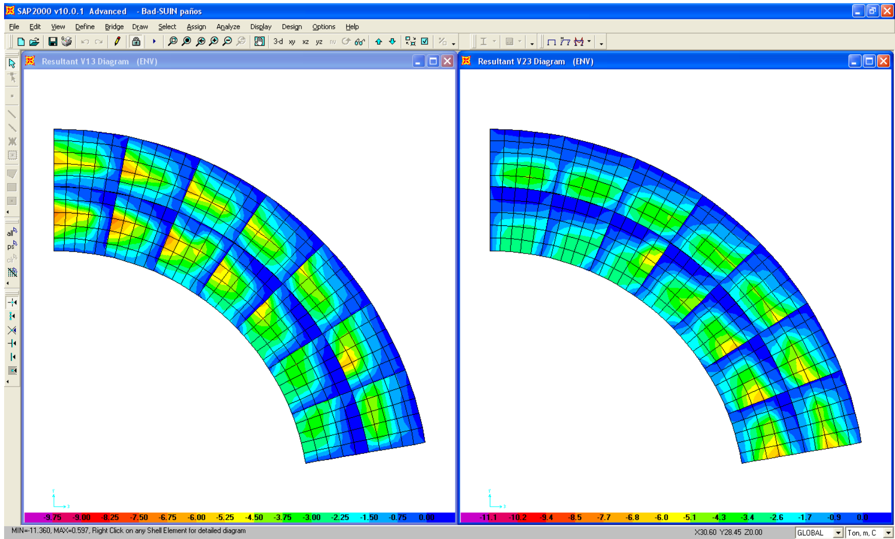
CORTANTES MIN. DIRECCIONES 1 Y 2
