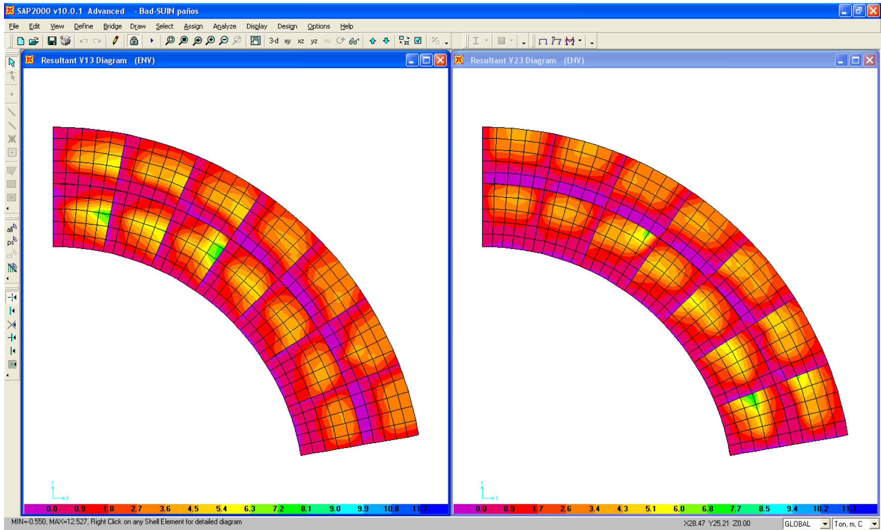
CORTANTES MAX. DIRECCIONES 1 Y 2
