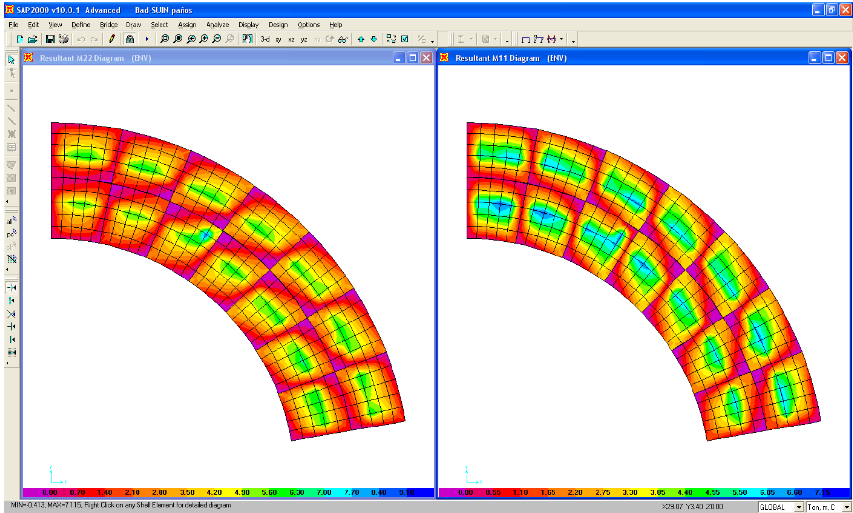
MOMENTOS MAX. DIRECCIONES 1 Y 2
