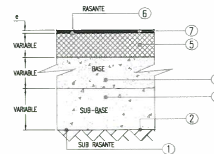
SECCION TIPICA DEL PAVIMENTO S/E
