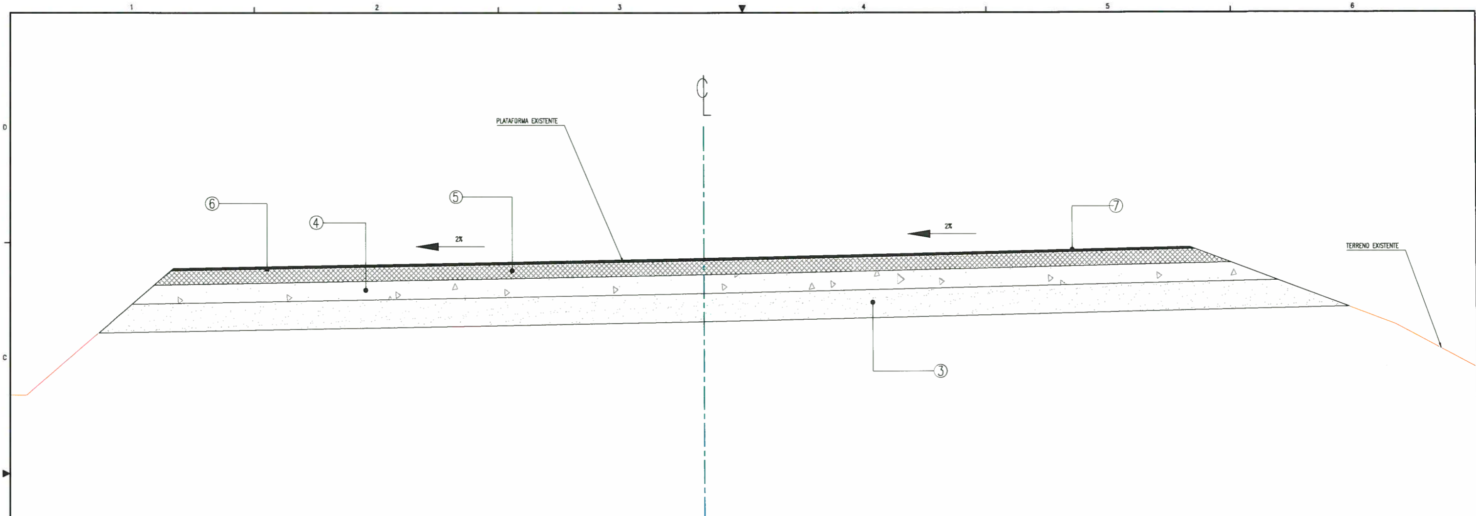
SECCION TIPICA EVITAMIENTO TRUJILLO
