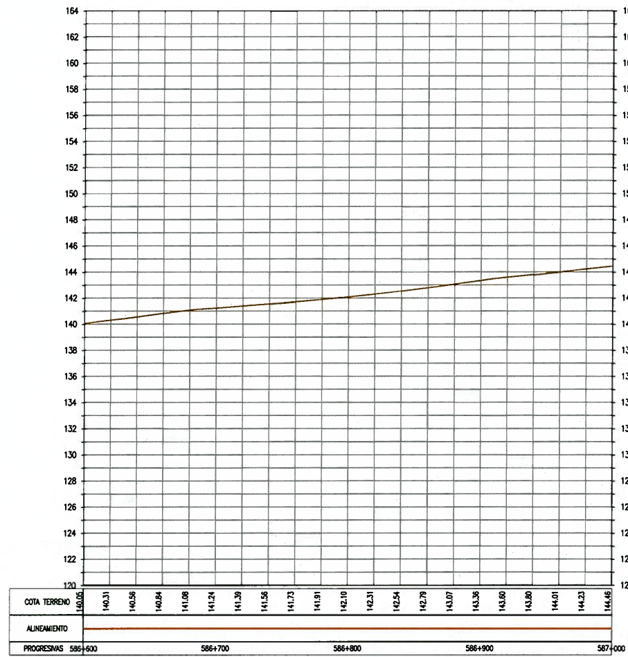
PERFIL LONGITUDINAL ESC H 1:2000, V 1:200
