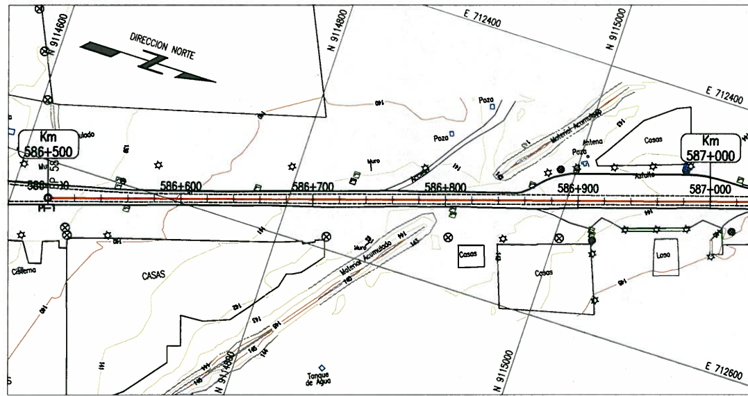
PLANTA ESC 1:2000
