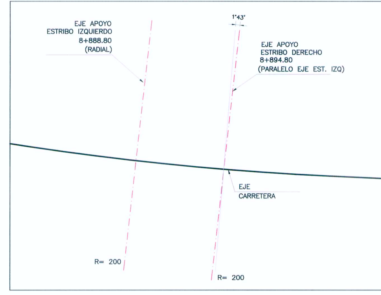
DETALLE TRAZO DE EJES Esc. 1/150
