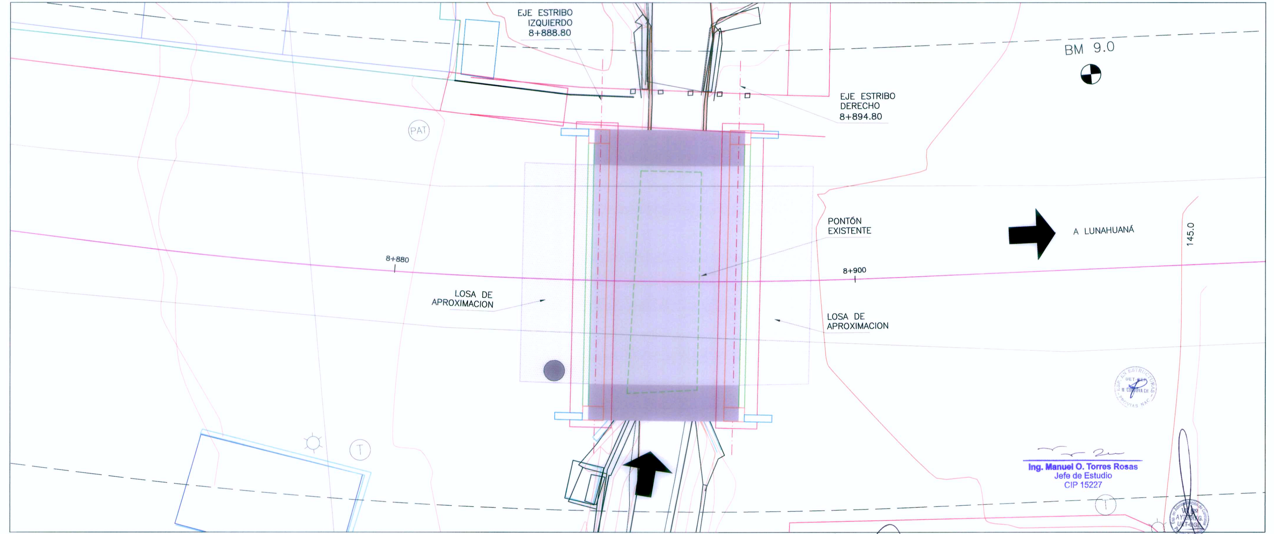
PLANTA Esc. 1/100
