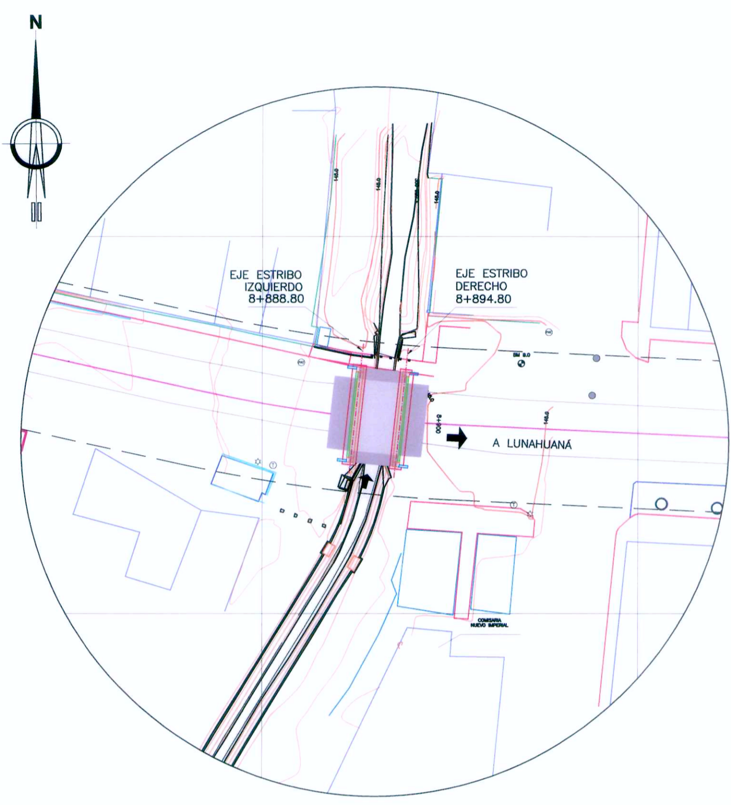
UBICACION Esc. 1/500
