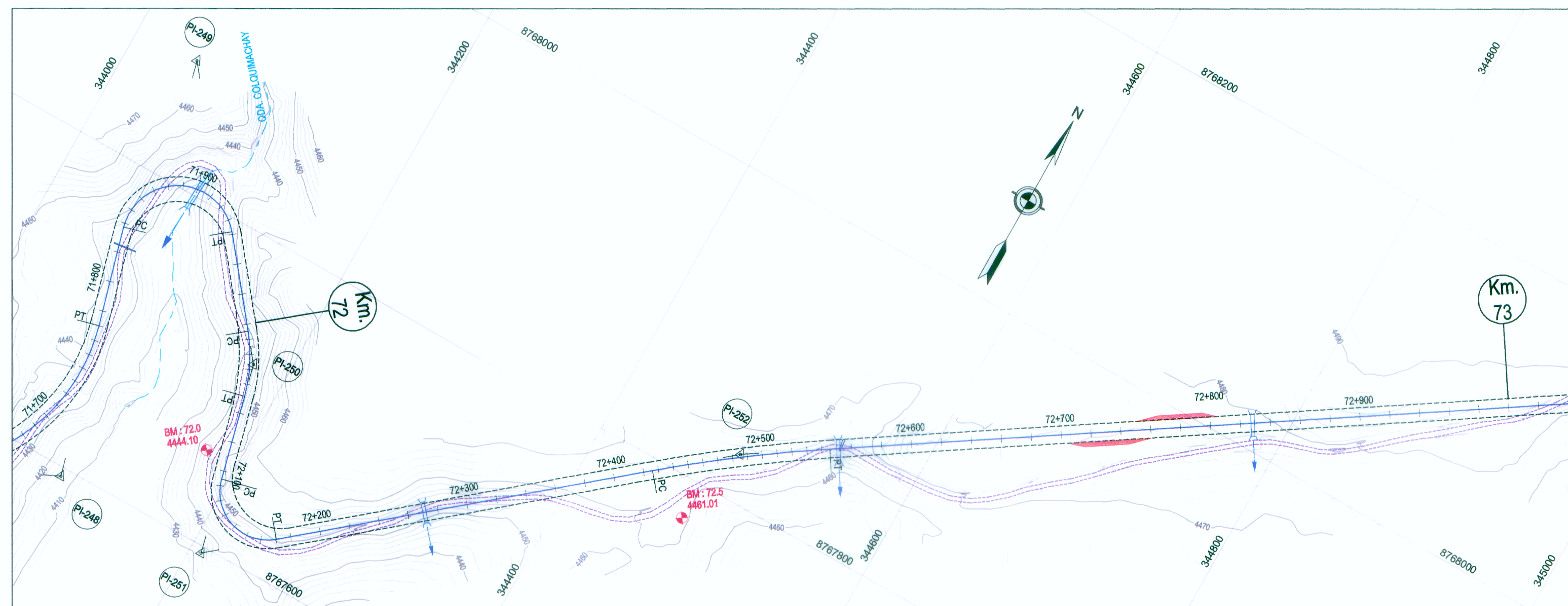
PLANTA H: 1/2,000
