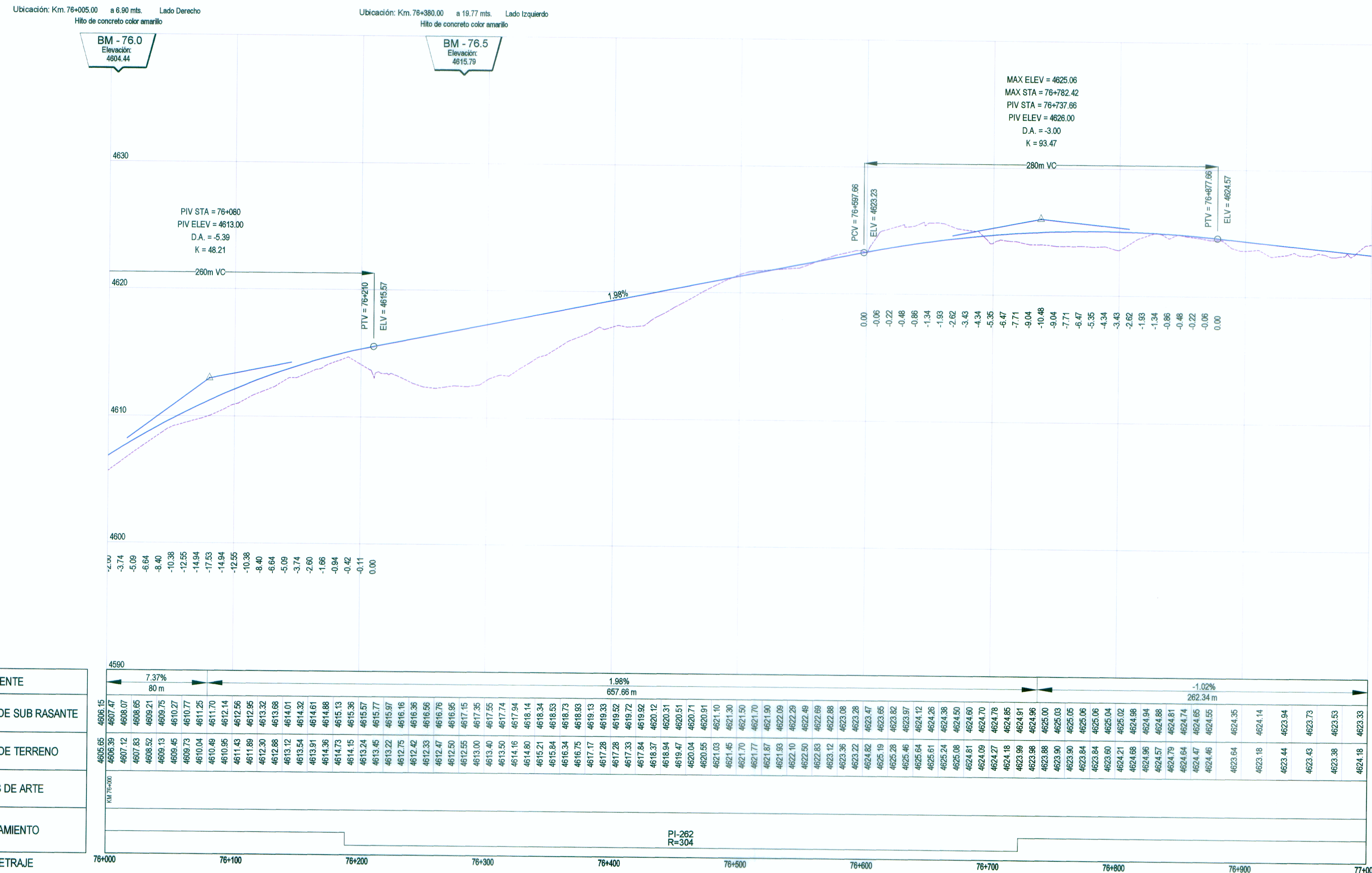
PERFIL LONGITUDINAL H: 1/2,000 V: 1/200
