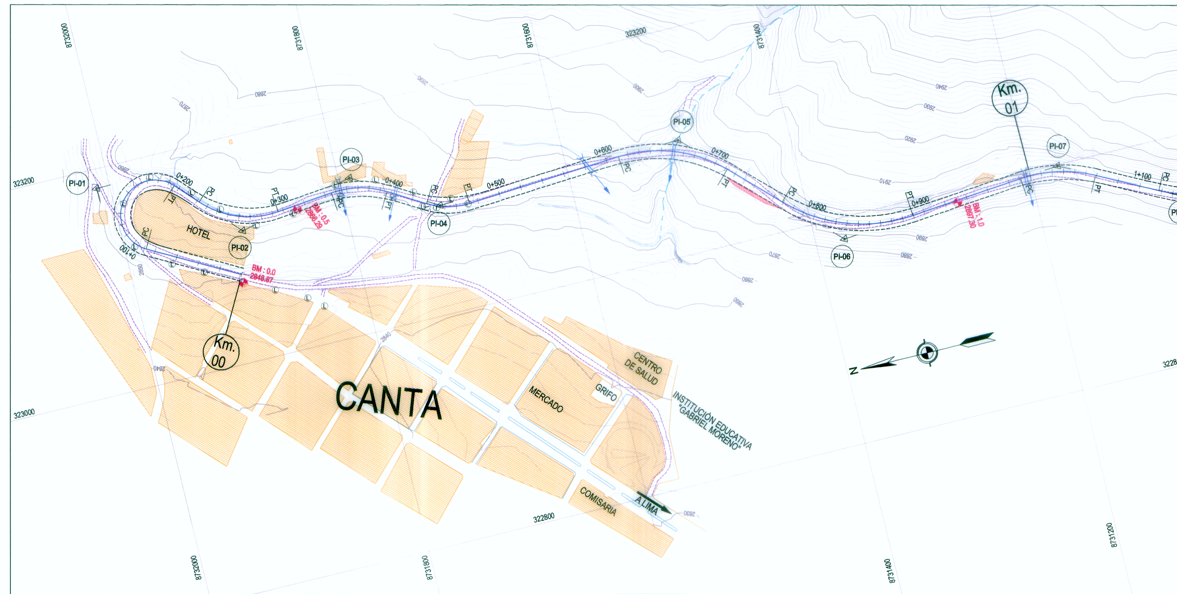
PLANTA H: 1/2,000
