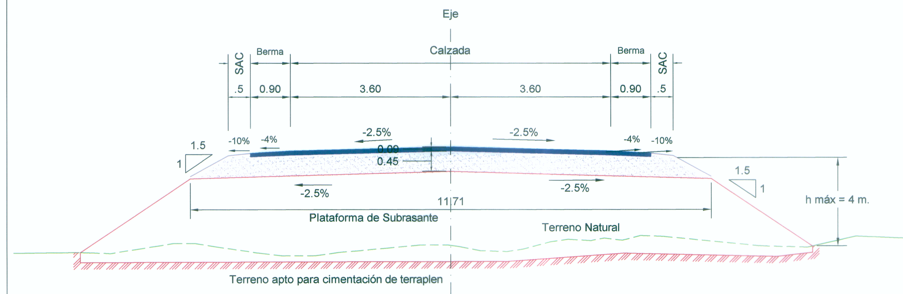
SECCIONES TÍPICAS EN TERRAPLEN (SIN BARRERAS DE SEGURIDAD)
