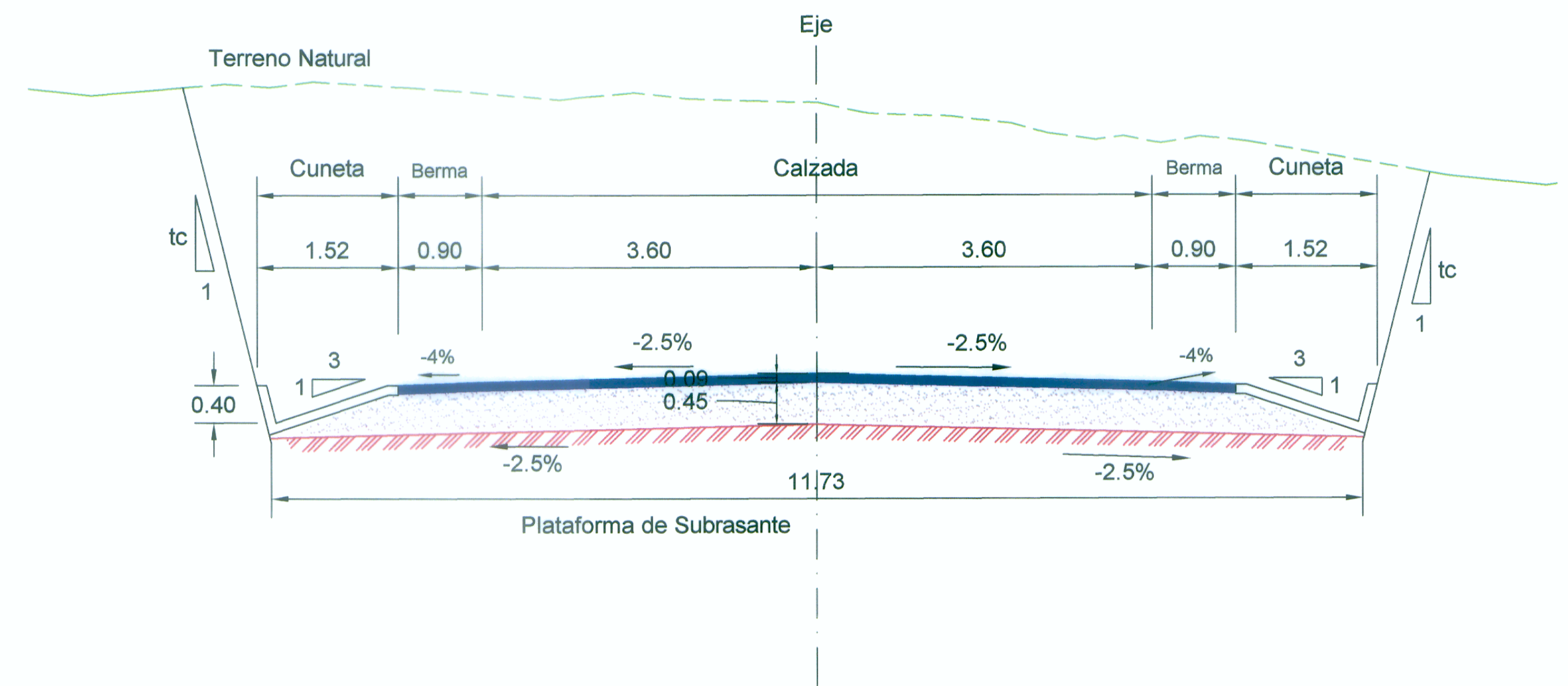
SECCIONES TÍPICAS EN CORTE CERRADO
