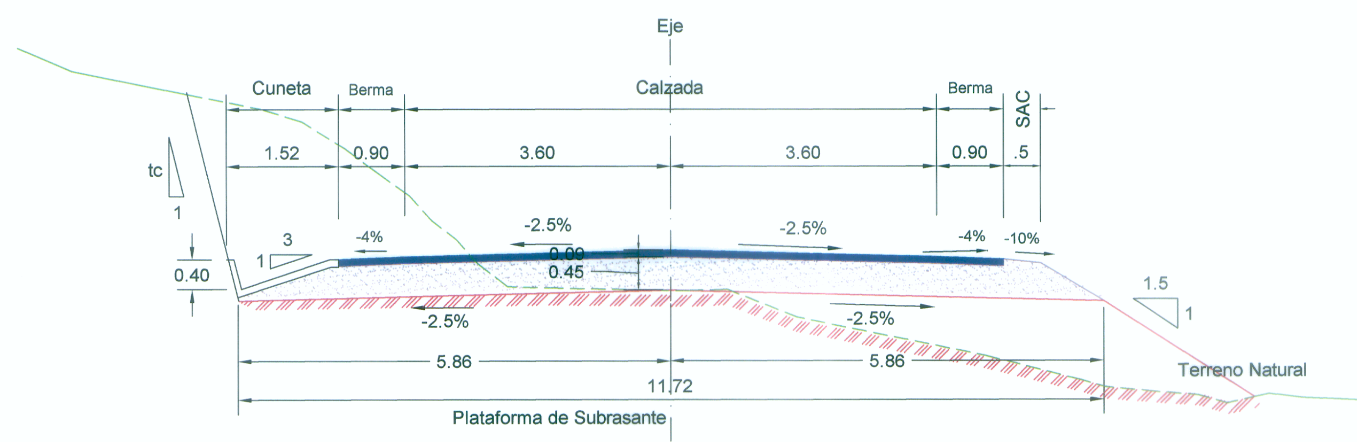
SECCIONES TÍPICAS A MEDIA LADERA
