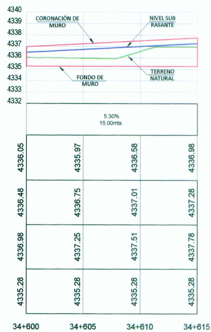
PERFIL LONGITUDINAL
