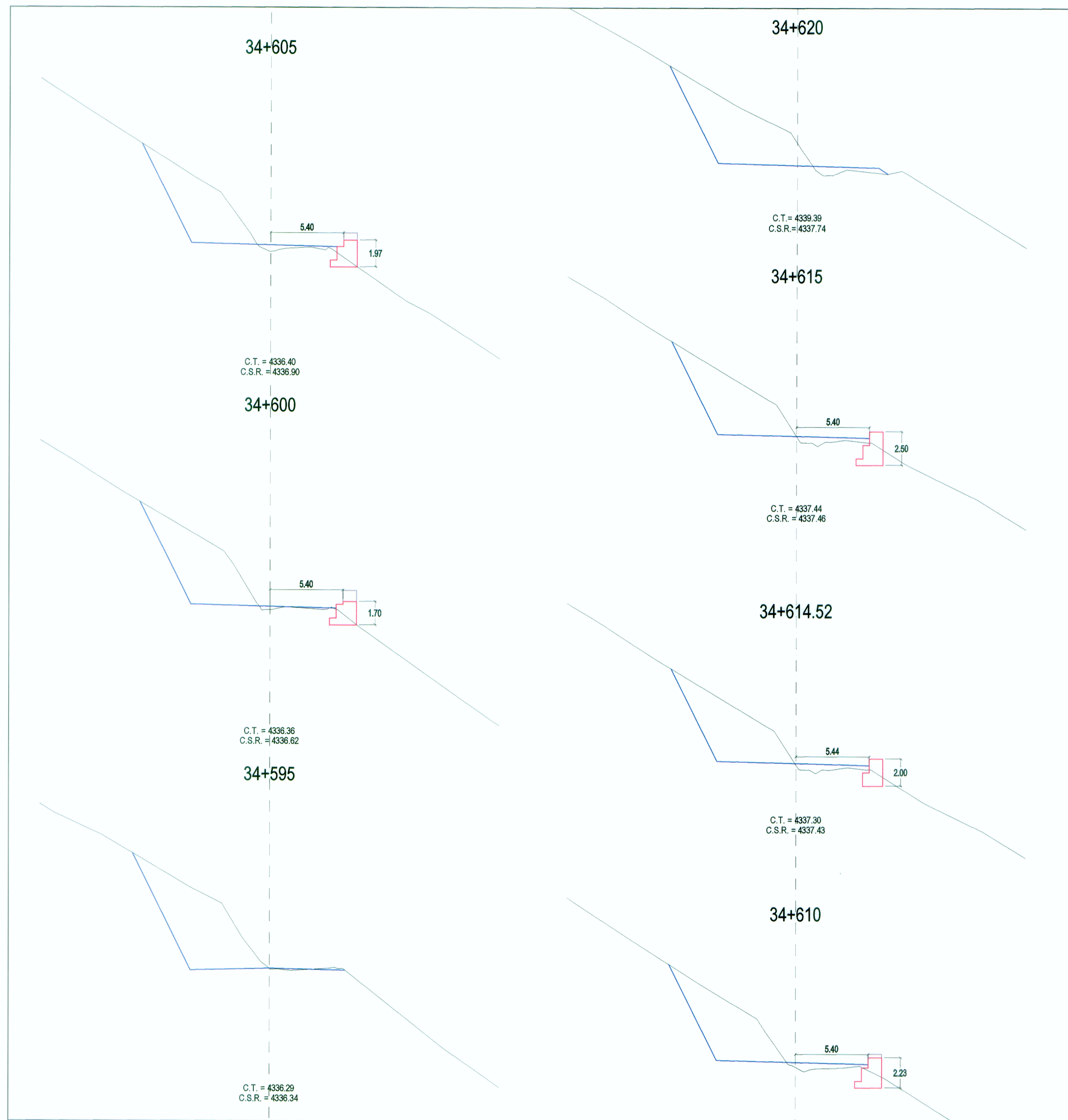
SECCIONES TRANSVERSALES
