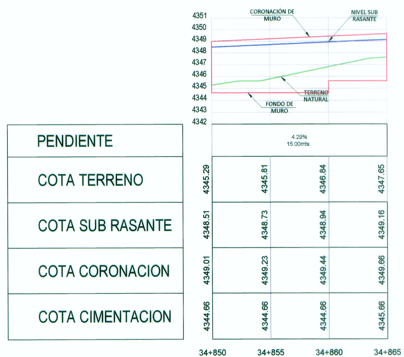
PERFIL LONGITUDINAL
