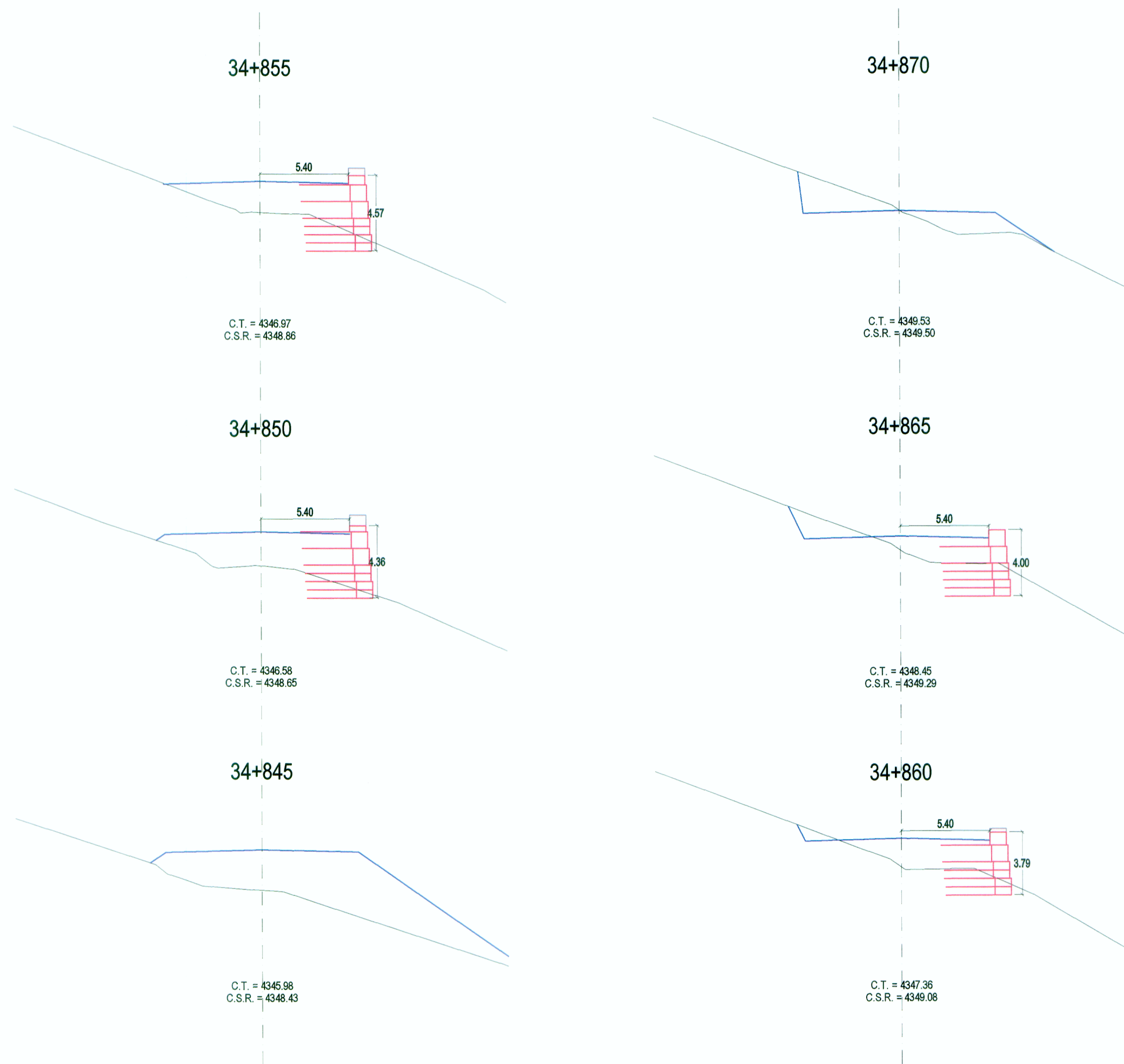
SECCIONES TRANSVERSALES
