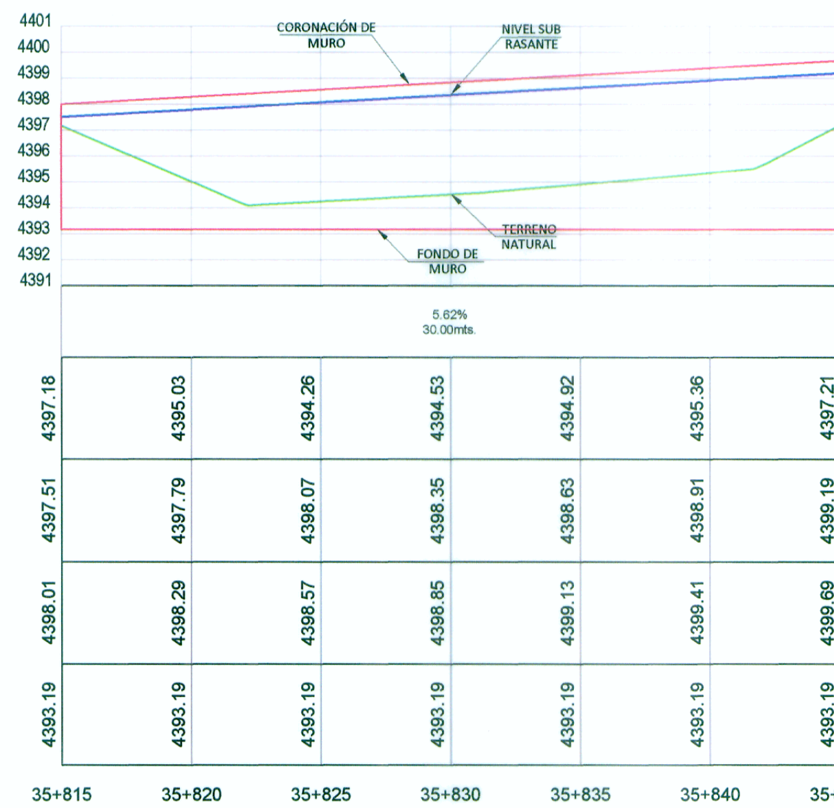
PERFIL LONGITUDINAL
