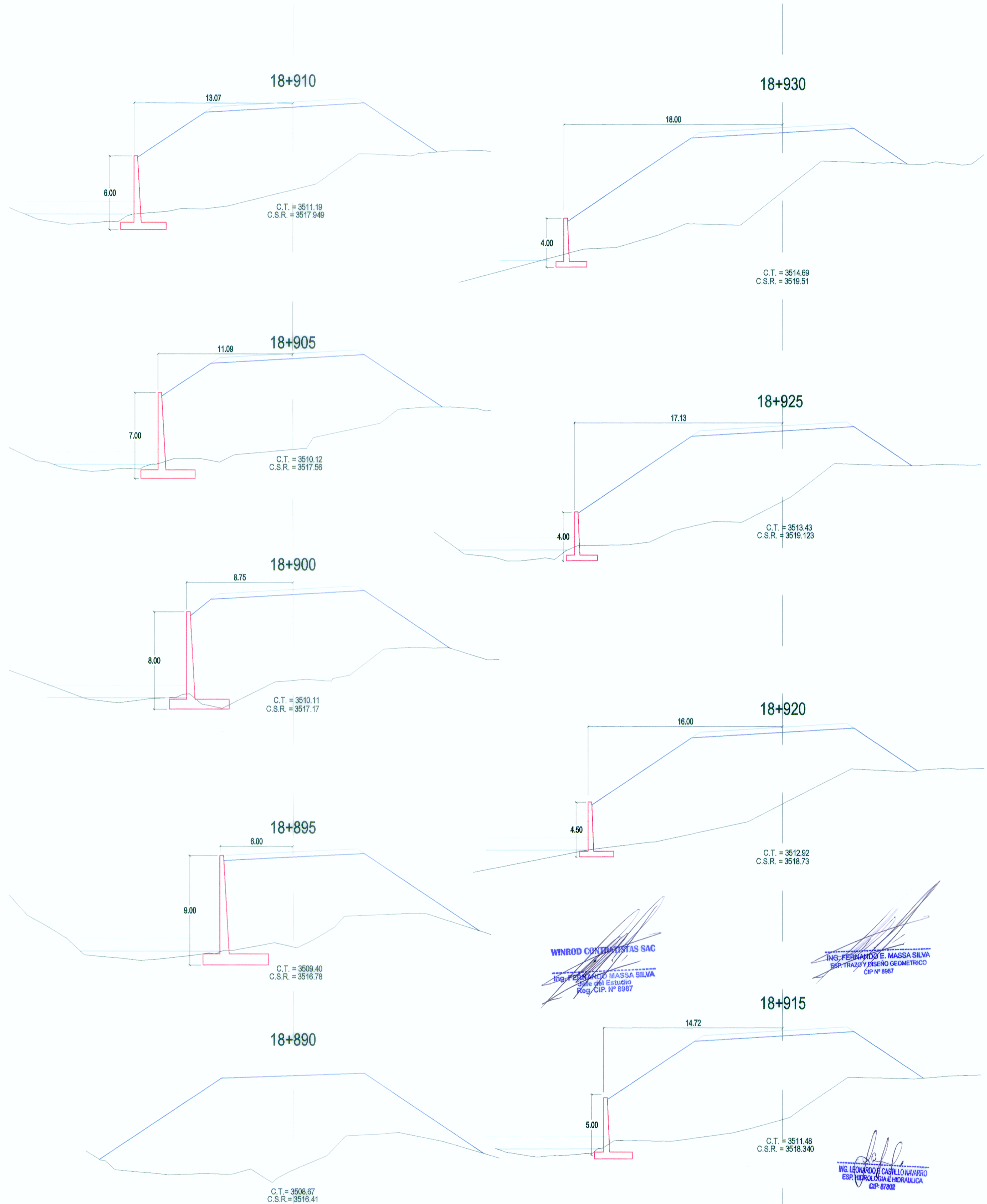
SECCIONES TRANSVERSALES
