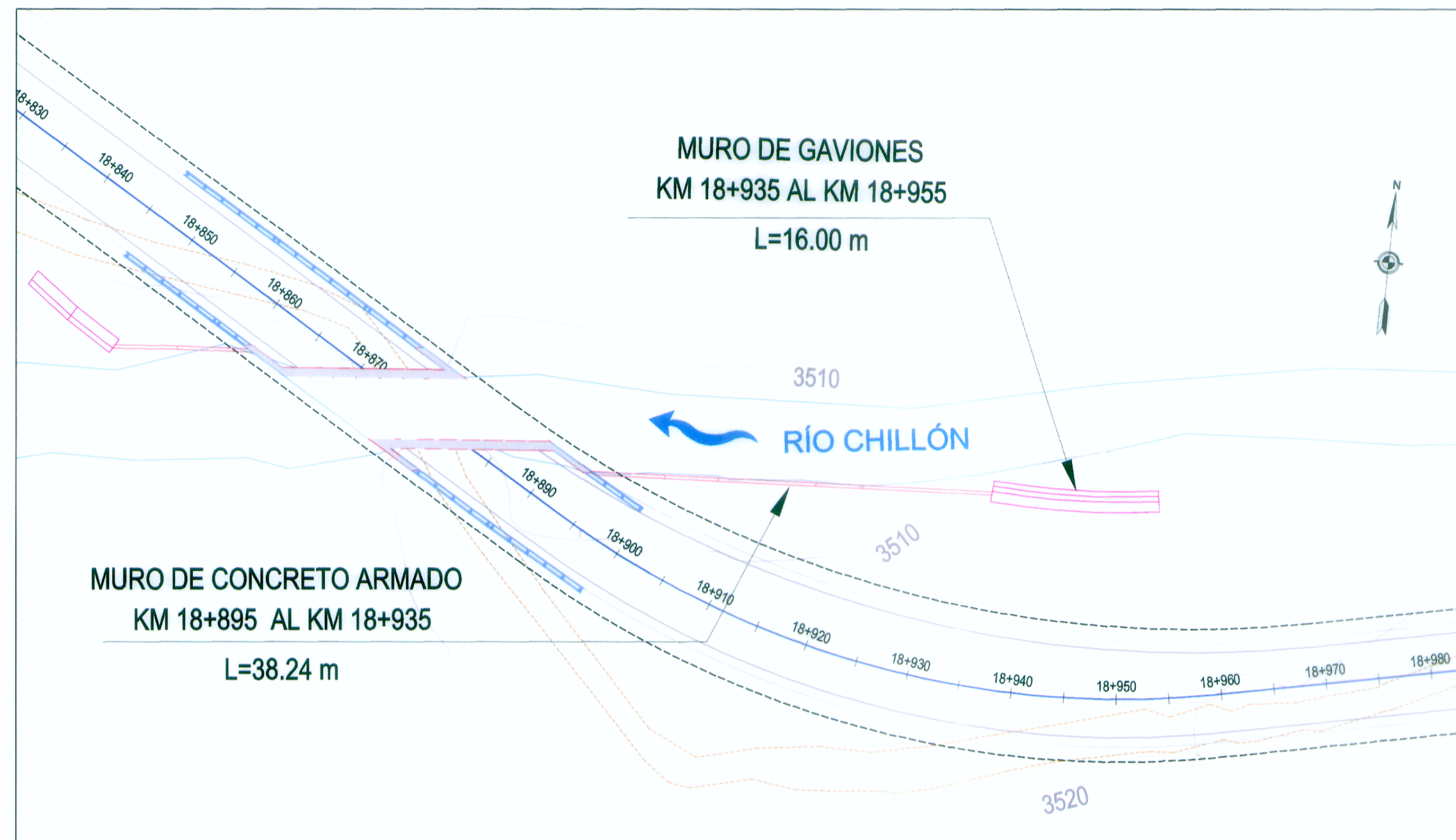
PLANTA
