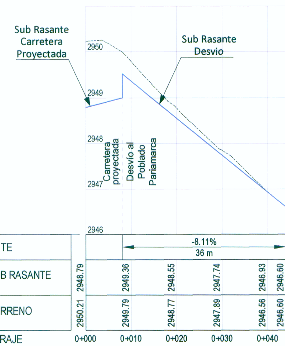
PERFIL LONGITUDINAL
