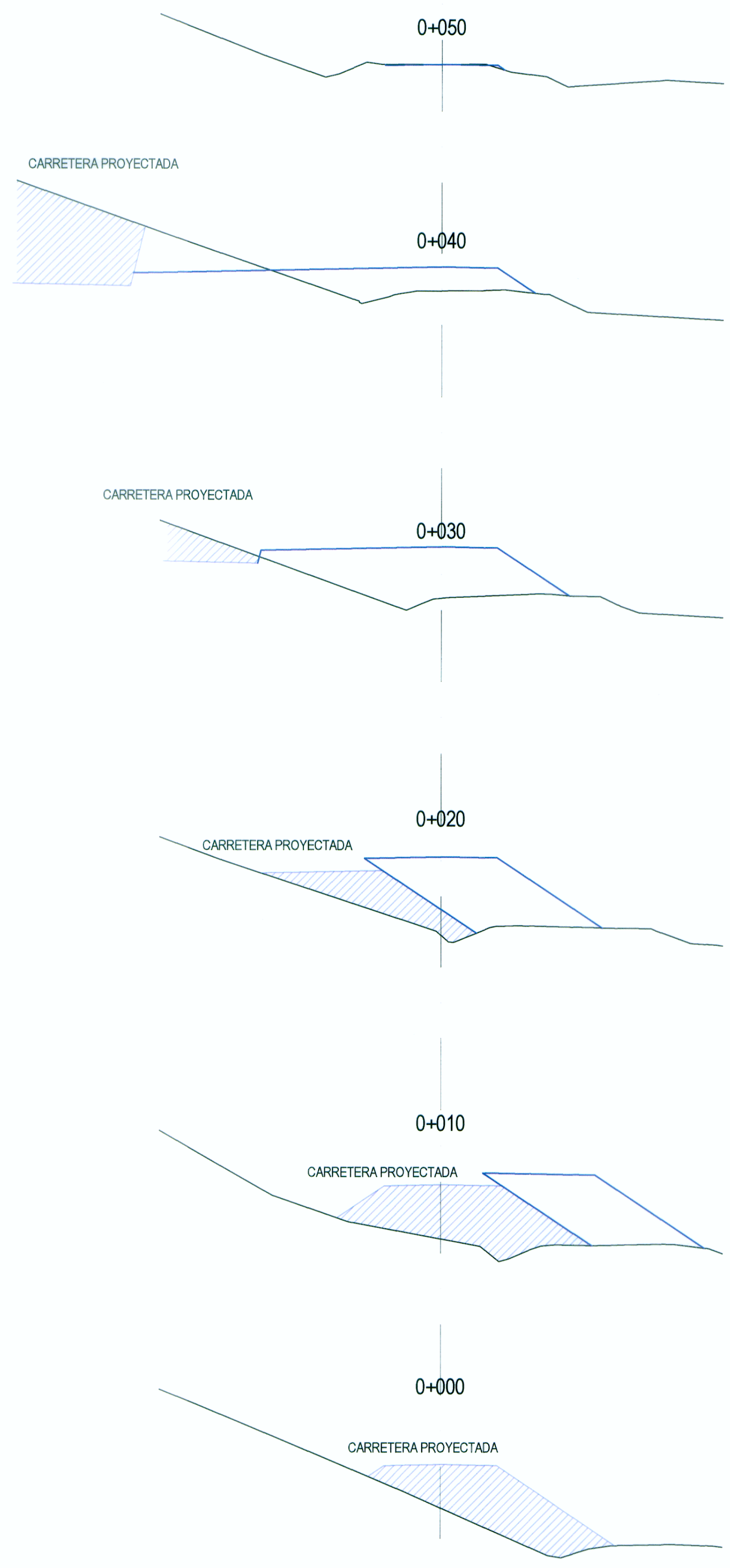
SECCIONES TRANSVERSALES ESC: 1/125
