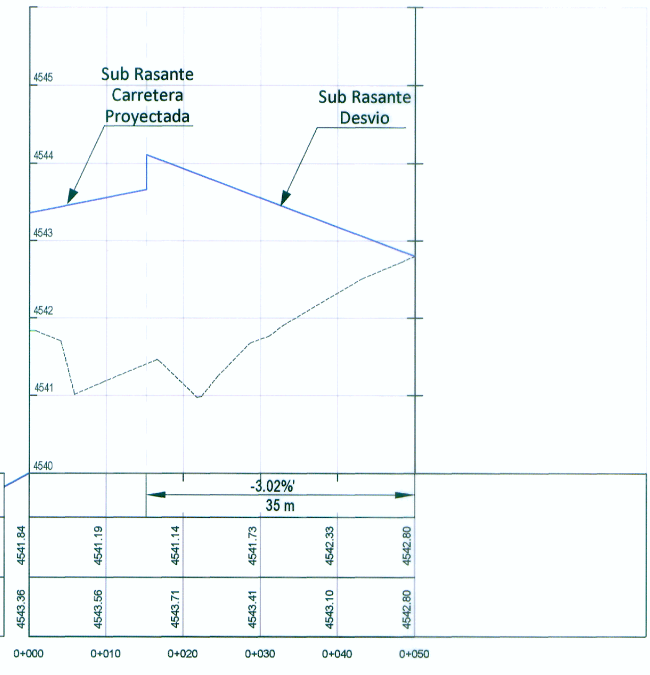
PERFIL LONGITUDINAL ESC: 1/500
