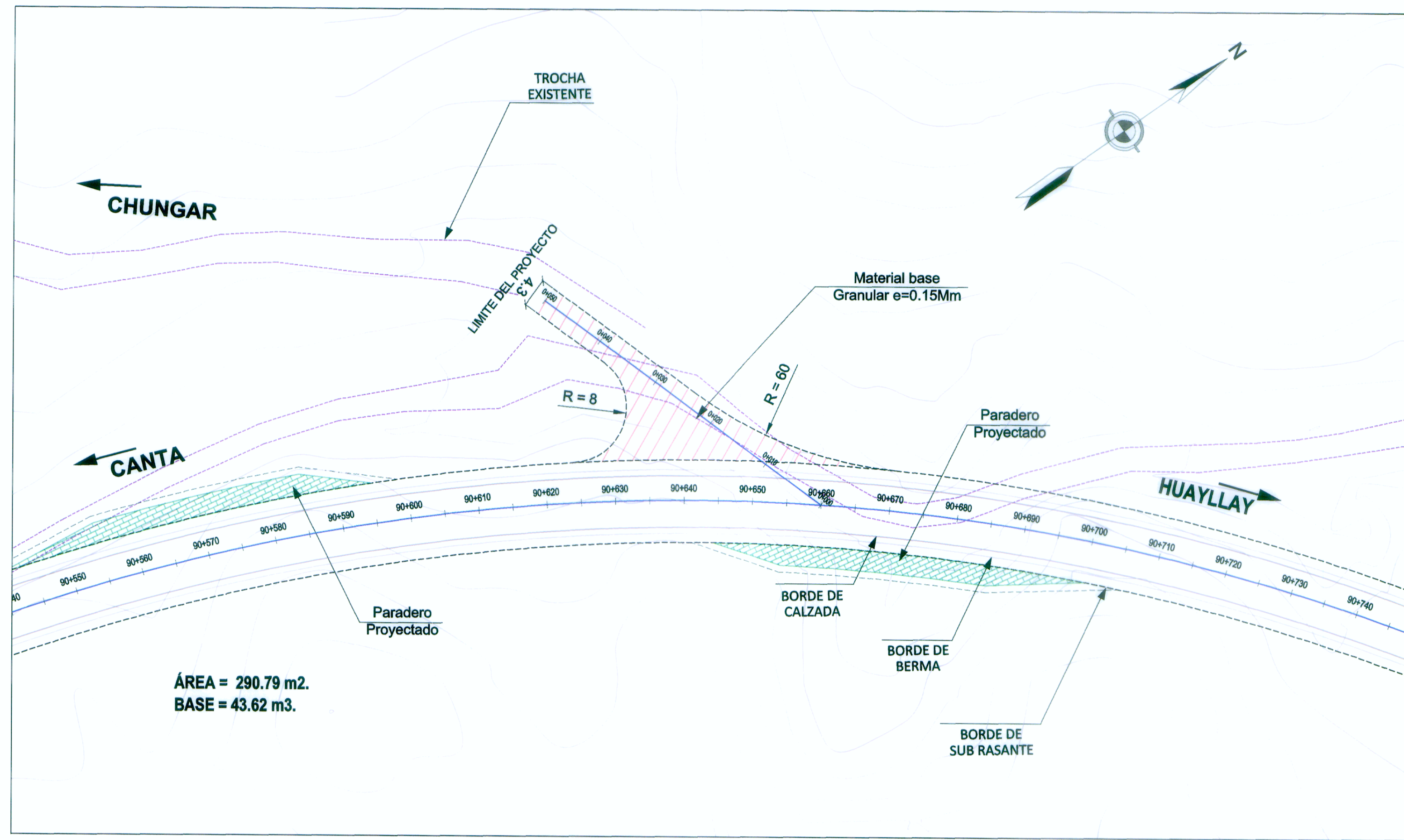
PLANTA ESC: 1/500
