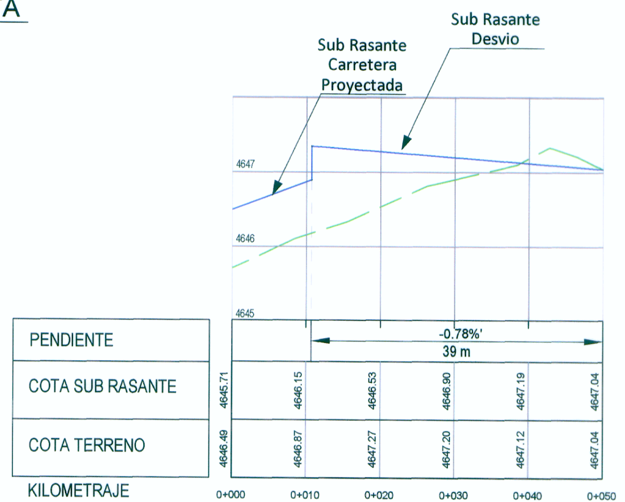
PERFIL LONGITUDINAL ESC: 1/500
