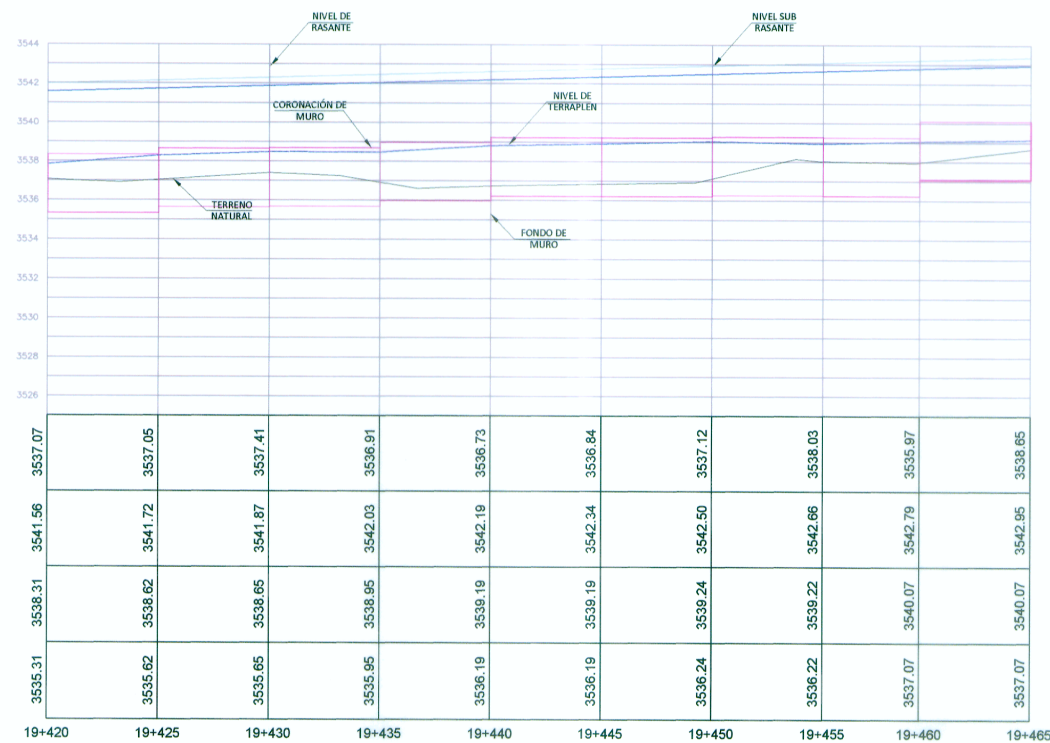
Muro Gavión 19+420 - 19+465
