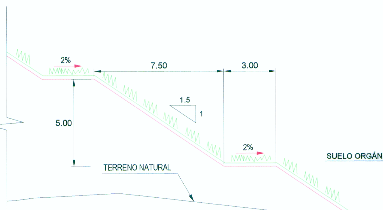
SECCIÓN TÍPICA DE BANQUETA
