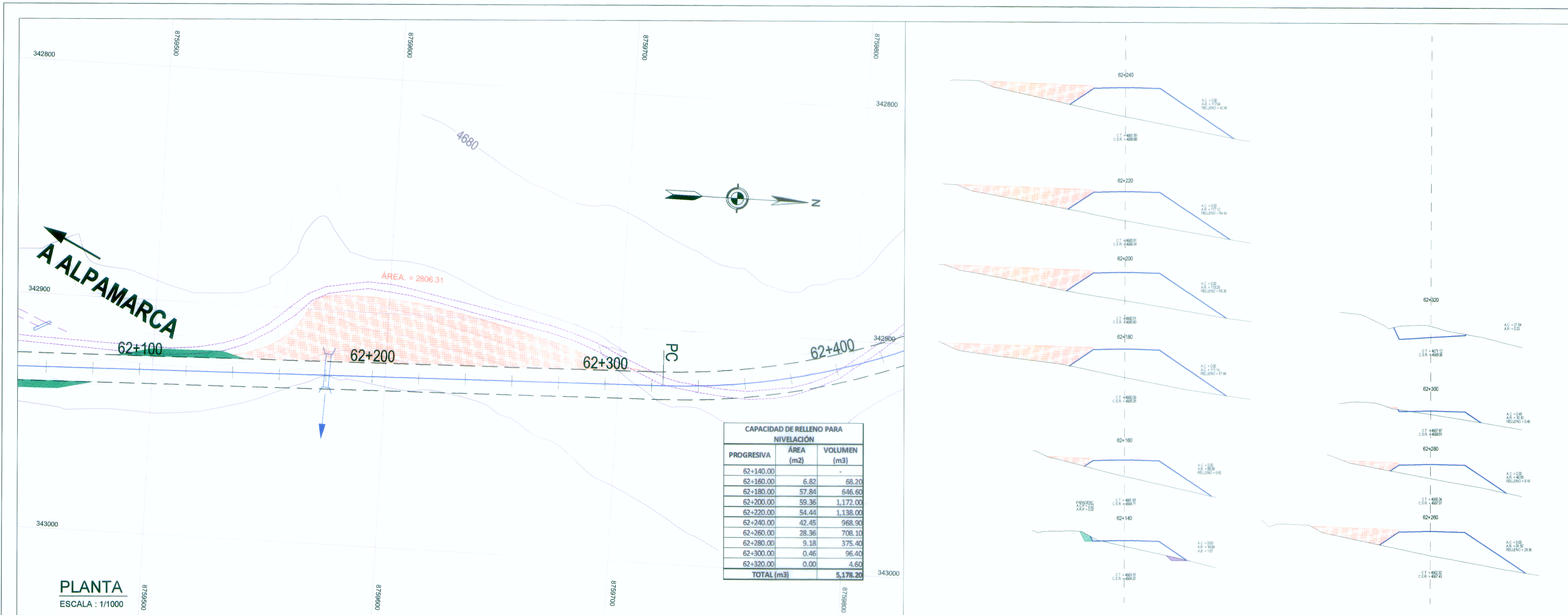
SECCIONES TRANSVERSALES ESCALA : 1/400
