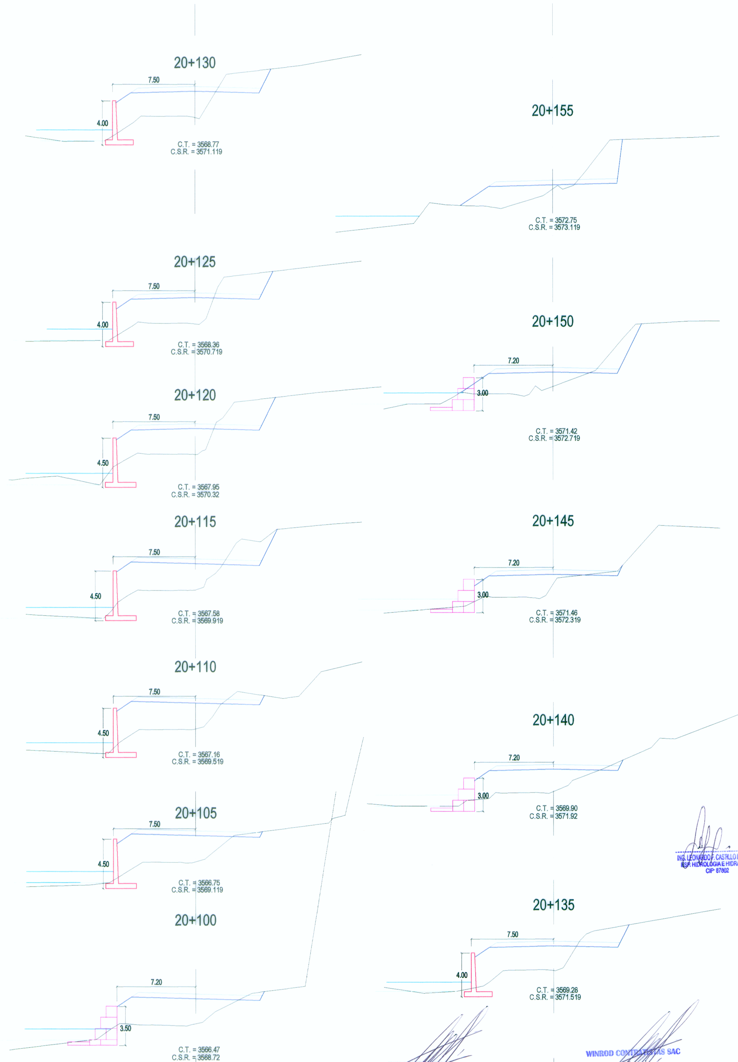
SECCIONES TRANSVERSALES
