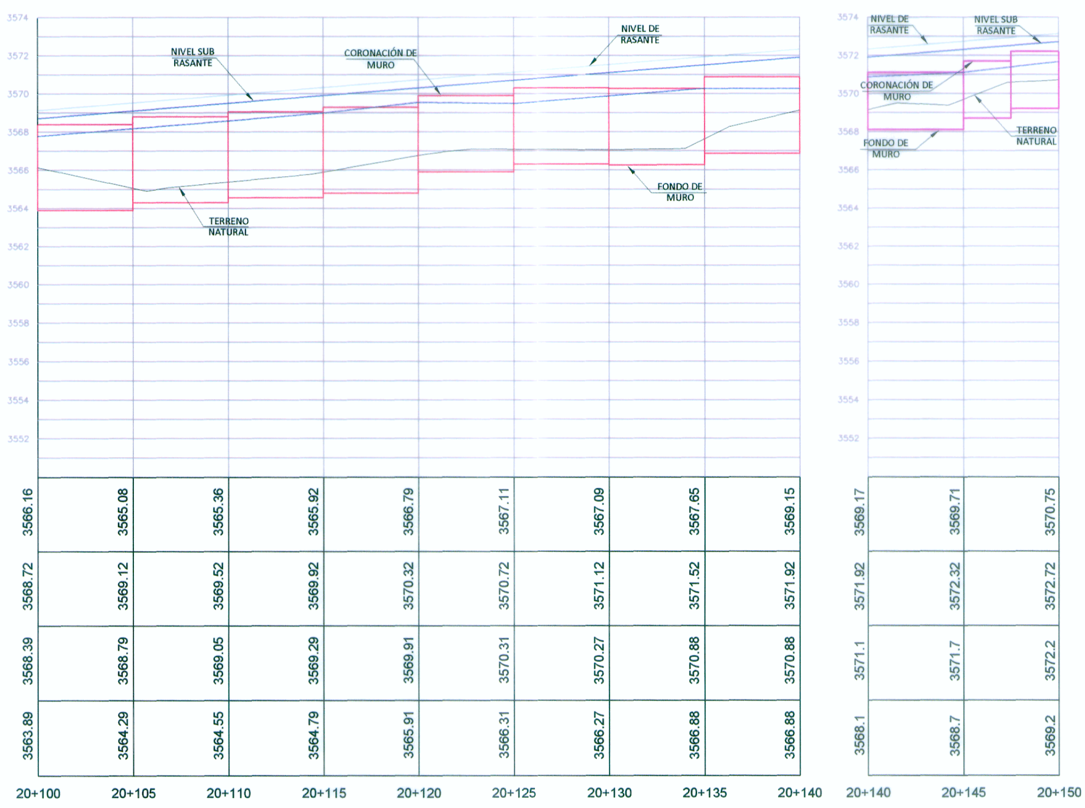
Muro Concreto y Muro Gavión 20+100 - 20+150
