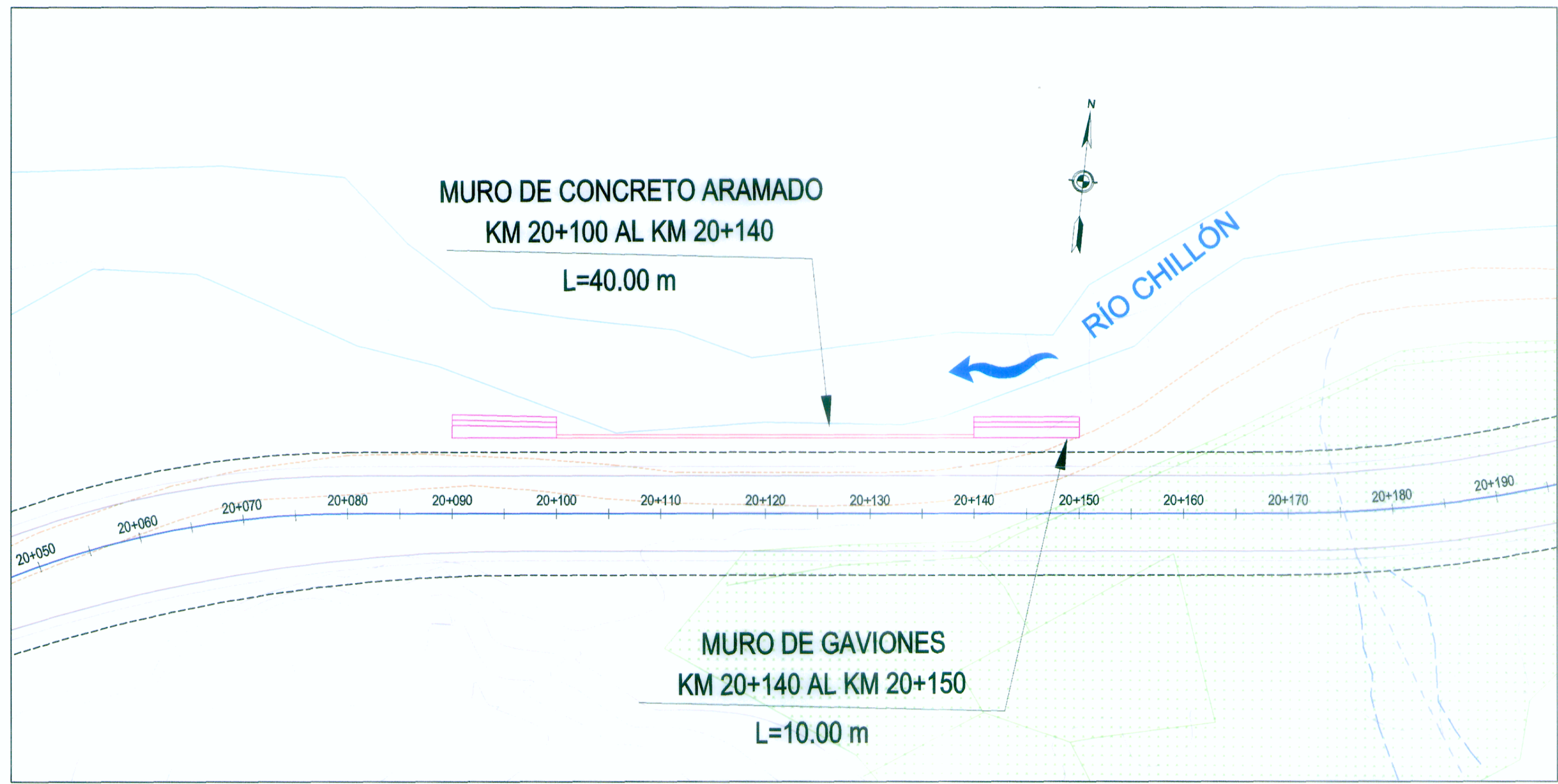
PLANTA
