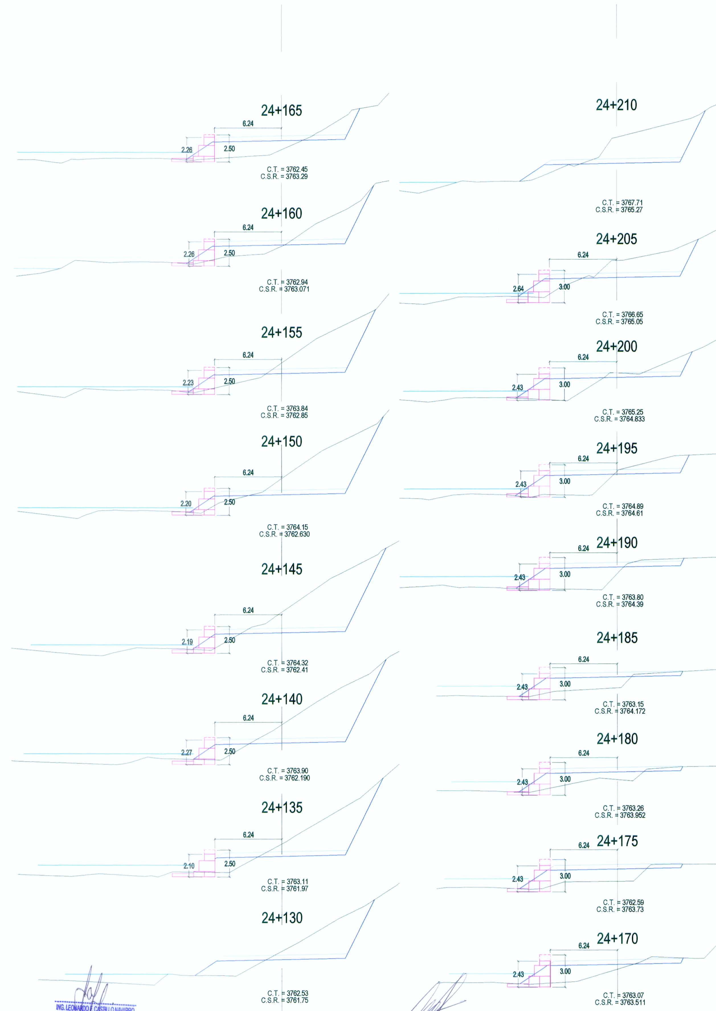
SECCIONES TRANSVERSALES Esc. 1/200
