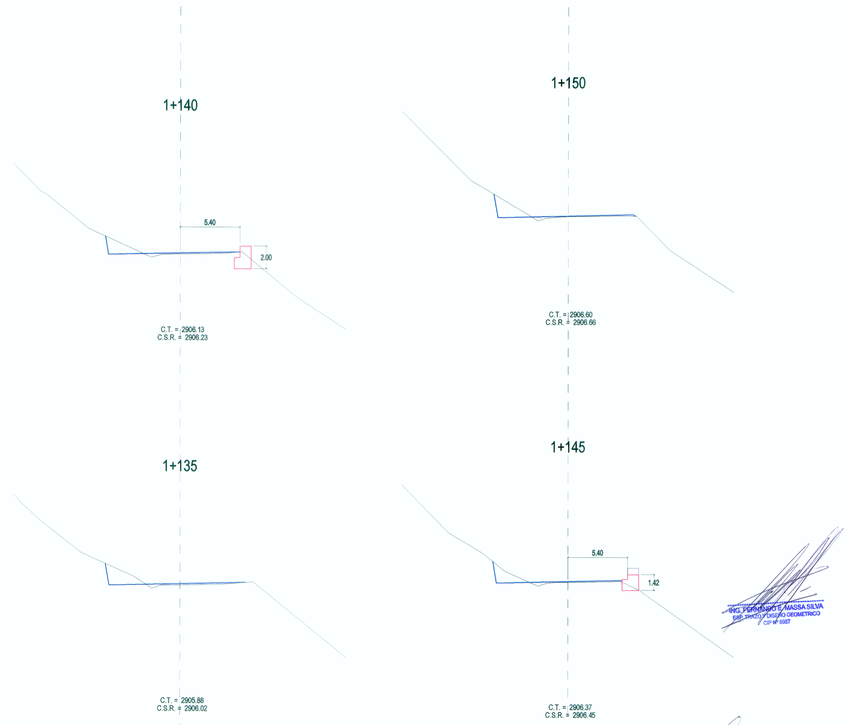
SECCIONES TRANSVERSALES
