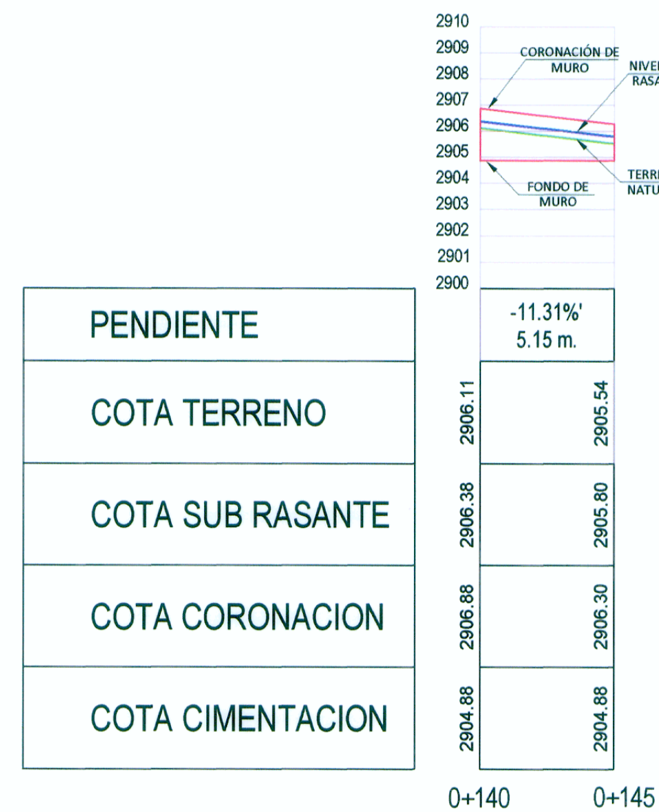
PERFIL LONGITUDINAL
