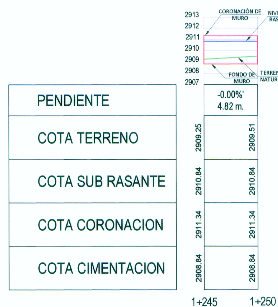
PERFIL LONGITUDINAL
