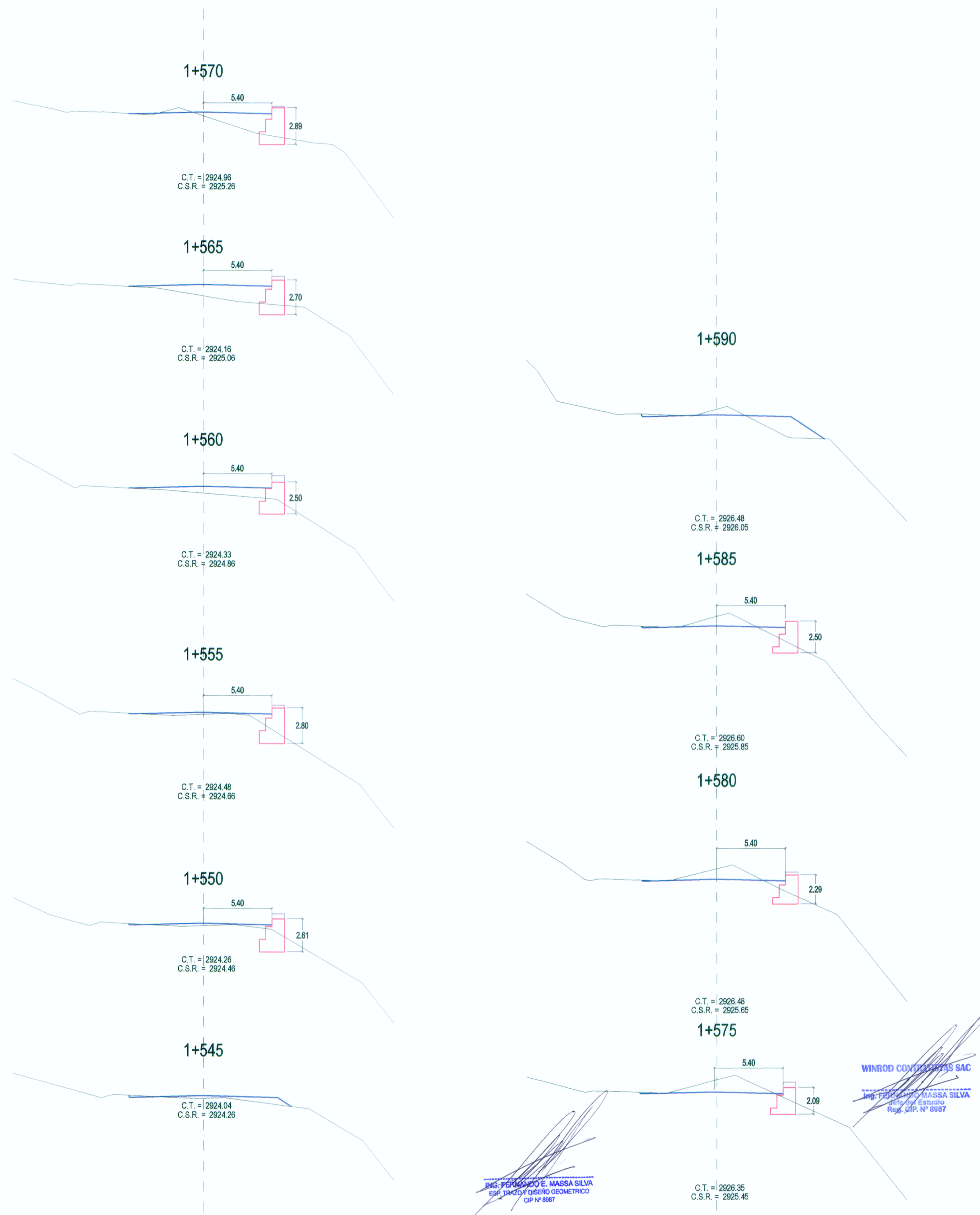
SECCIONES TRANSVERSALES
