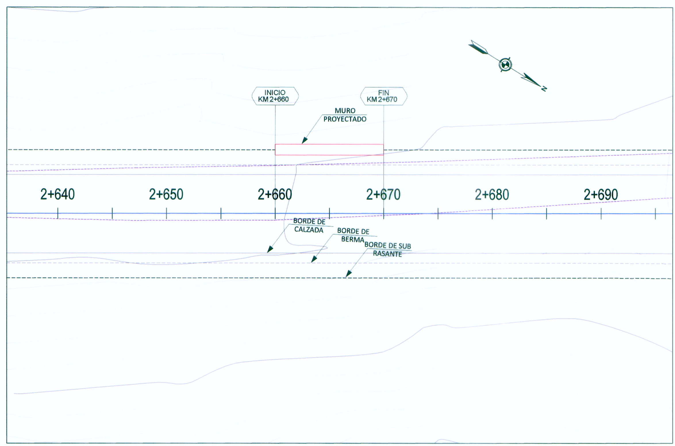
PLANTA
