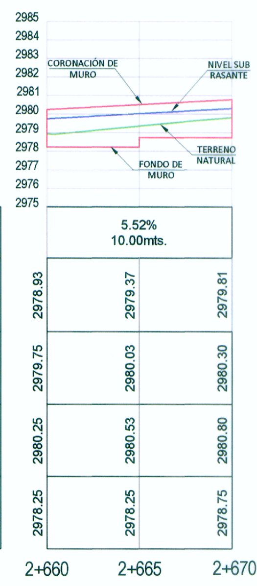
PERFIL LONGITUDINAL
